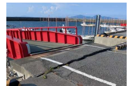
漁港の被害 （浮桟橋接続部のクラック）
