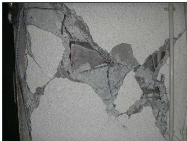
【鉄筋コンクリート造】 鉄筋が大きく露出しており、鉄筋の曲がり・破断が見られる。
