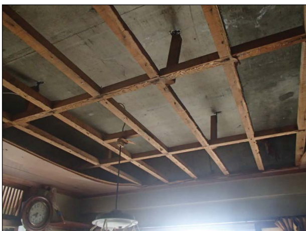
【天井】 天井板が脱落している。
