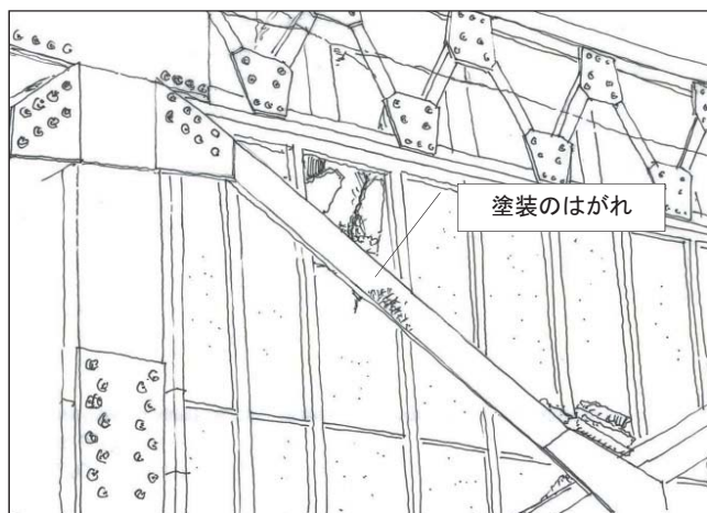
【鉄骨造】 わずかな座屈変形が見られる。 50022
