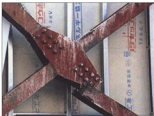
【鉄骨造】 破断が見られる。 50024
