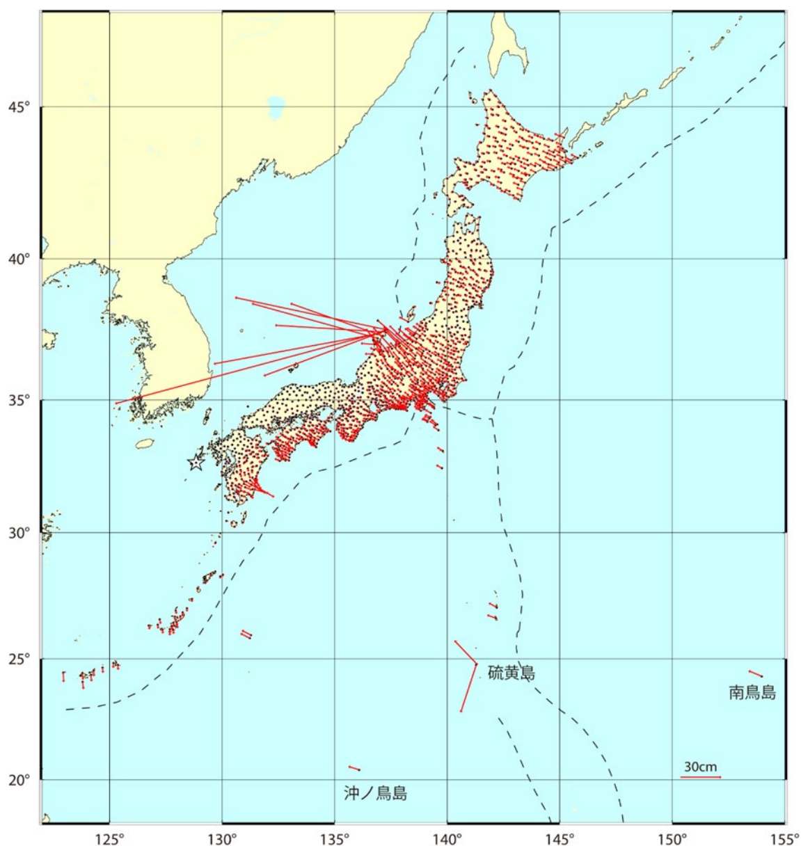
図 GNSS による全国水平地殻変動図（2023 年 9 月～2024 年 9 月）
