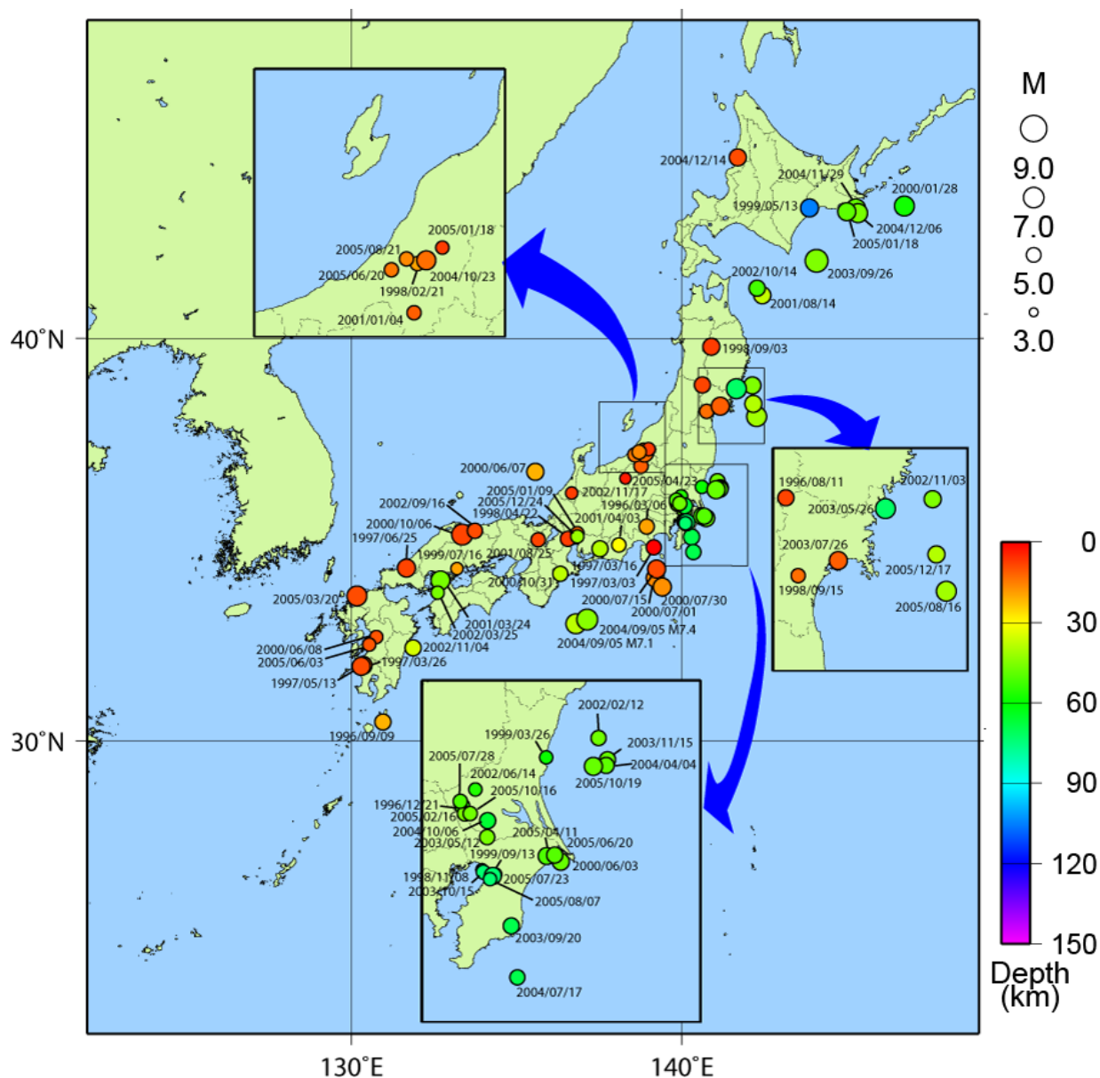
図 日本付近で発生した主な被害地震の震央分布（平成8年～平成17年）
