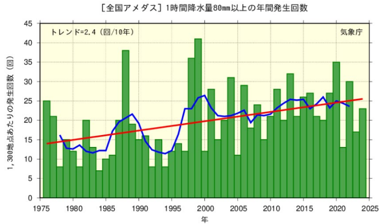
図 1 1時間降水量 80 ミリ以上の年間発生回数 (1976 年から 2024 年)
