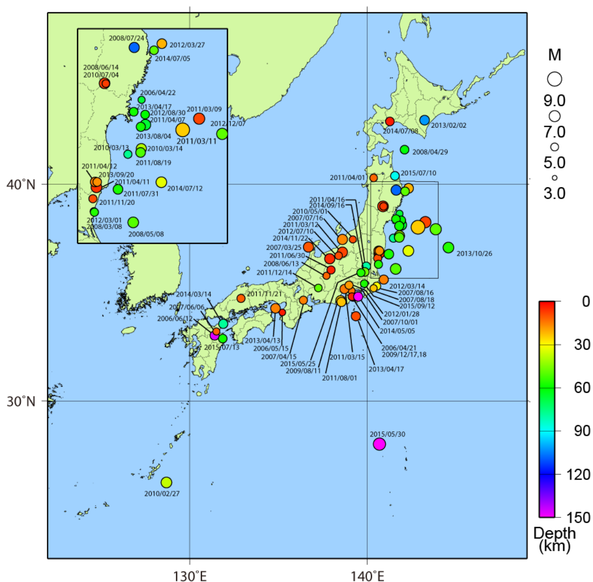
図 日本付近で発生した主な被害地震の震央分布（平成 18 年～平成 27 年）
