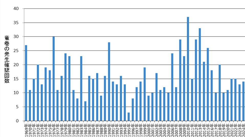
図 竜巻発生確認回数の推移
