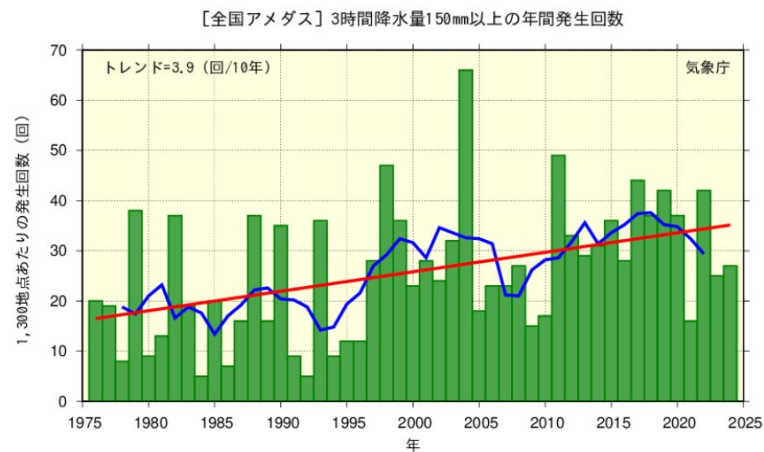
図 3 3時間降水量 150 ミリ以上の年間発生回数 (1976 年から 2024 年)
