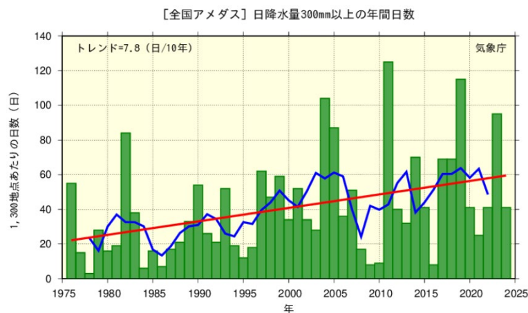
図 日降水量 300 ミリ以上の年間発生回数 (1976 年から 2024 年)
