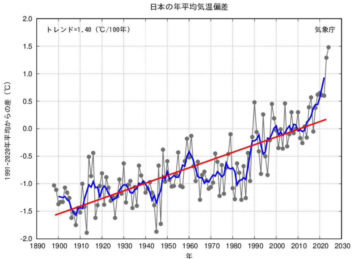
図 日本の年平均気温偏差
