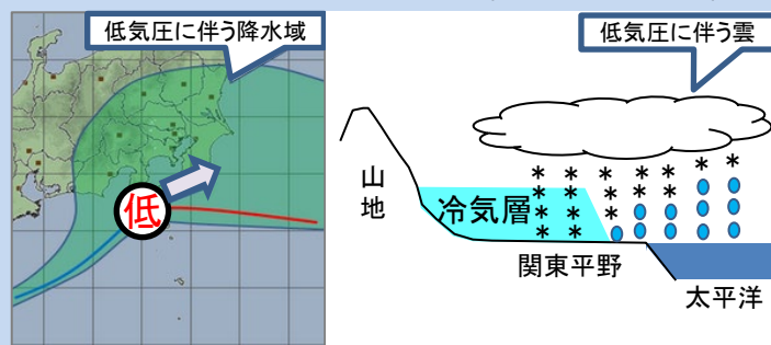
南岸低気圧による降雪の概念図(関東地方の場合)
