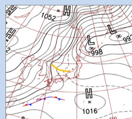
里雪型の天気図と概念図
