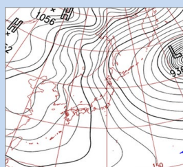
山雪型の天気図と概念図
