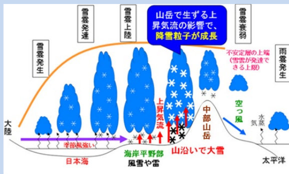
山雪型の天気図と概念図
