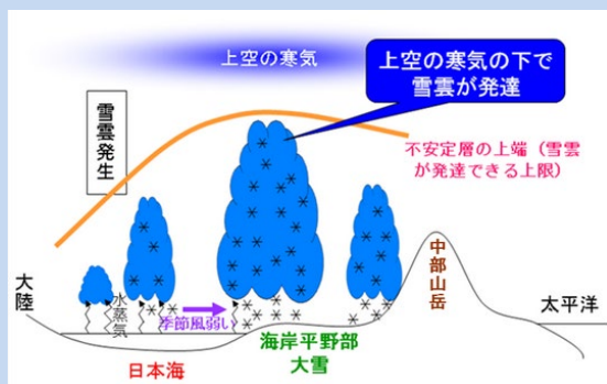
里雪型の天気図と概念図
