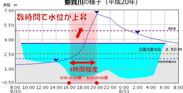
平成28年8月台風第10号災害時の小本川の水面上昇
