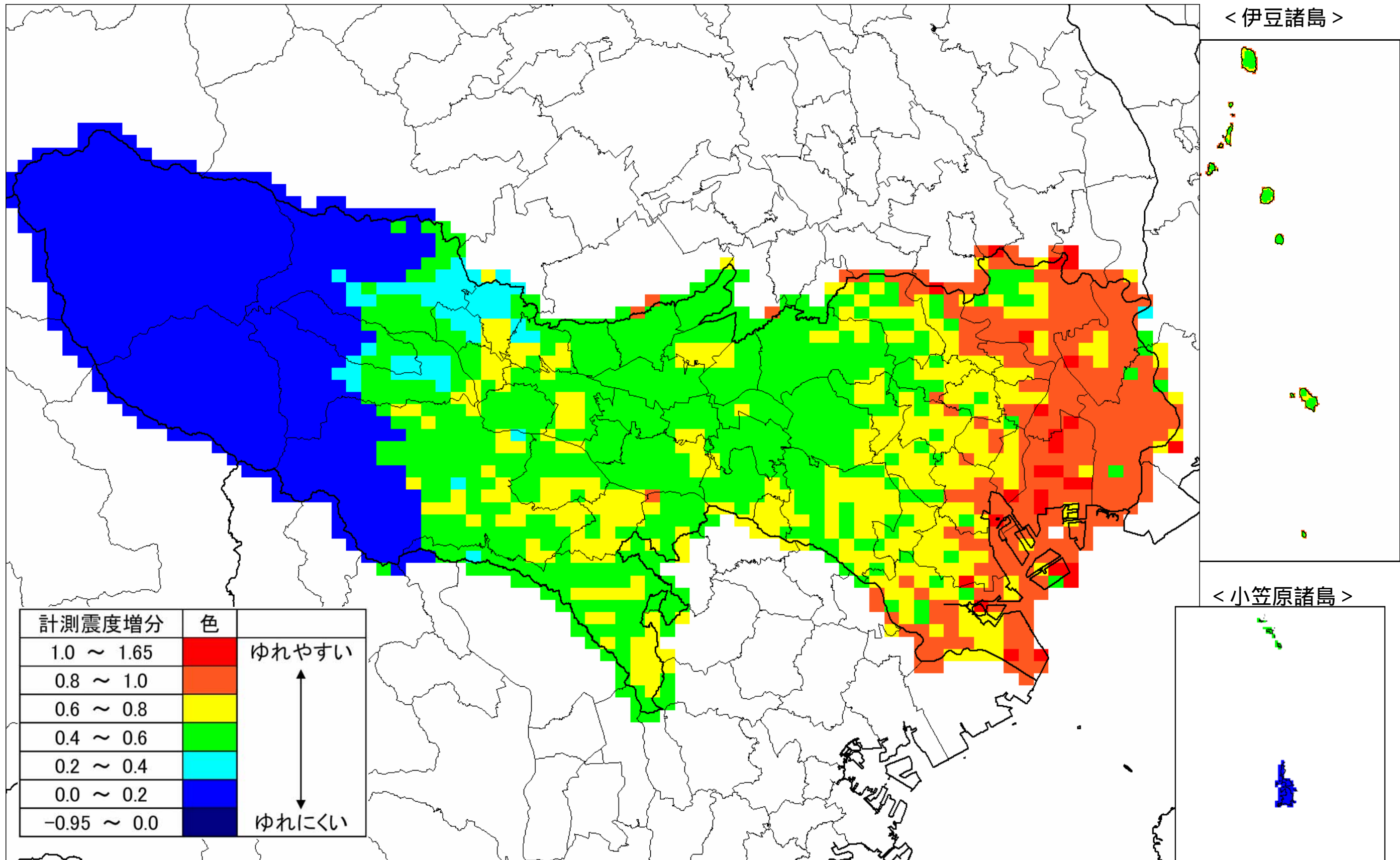
図 表層地盤のゆれやすさ（東京都）
