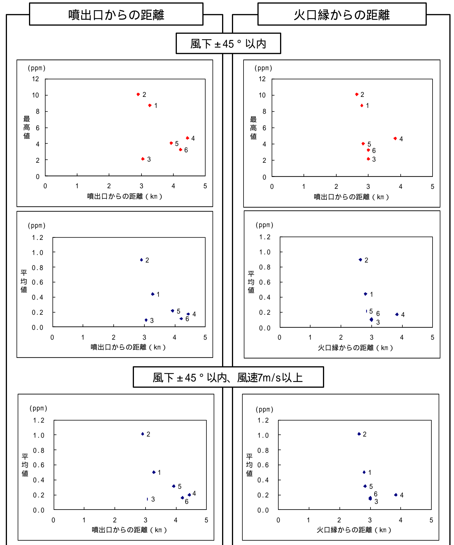
図16 噴出口および火口縁からの距離と濃度 (1時間値、山麓)
