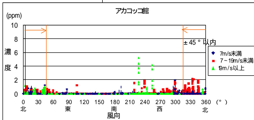
図11 風向・風速別濃度分布 (1時間値)
