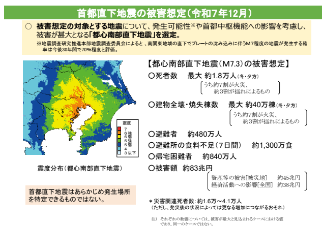
図1 新たな首都直下地震の被害想定
