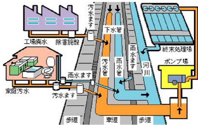
下水道施設の構成
