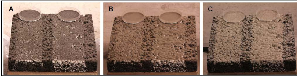
A: 玄武岩、B: 安山岩、C: 流紋岩質の火山灰(中粒:最頻粒径200-260 \mu\text{m} )により、路面標示が8%以下となったときの平均厚さの実験(Blake et al. 2016a)。
