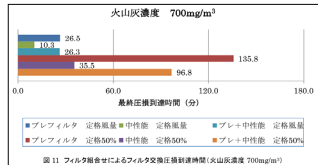
図 11 フィルタ組合せによるフィルタ交換圧損到達時間(火山灰濃度 700mg/m 3 )
