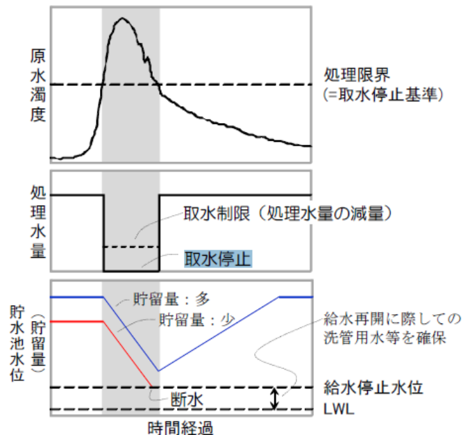
濁度による取水停止イメージ
