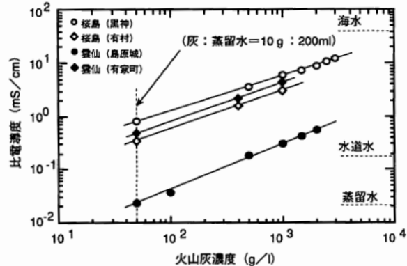
火山灰濃度と比電導度の関係 (川畑・他, 1995)
