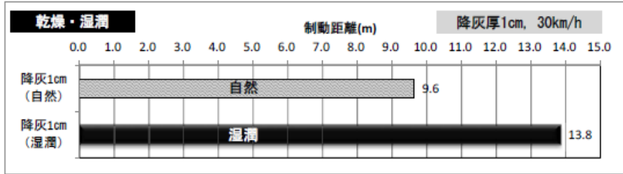
図 4-2 制動距離試験結果（降灰厚 1 cm 時速 30 km/h）
