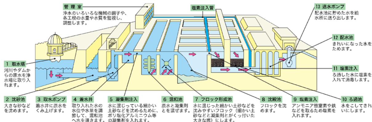
一般的な浄水の仕組み（急速ろ過法）
