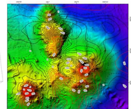
海徳海山全磁力異常図
