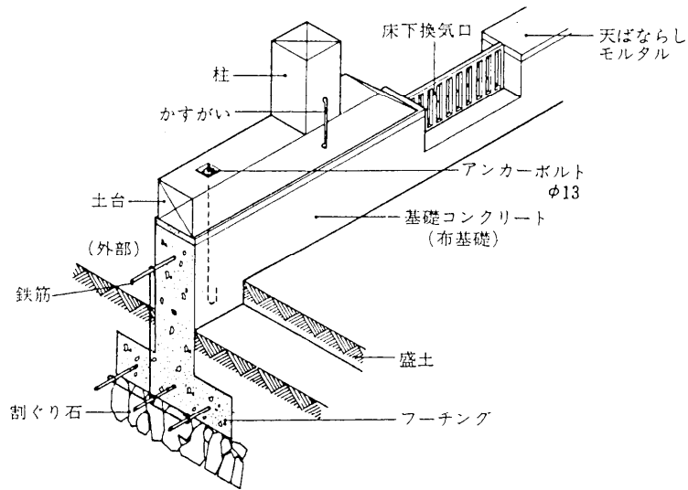
布基礎
