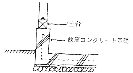
ベタ基礎
