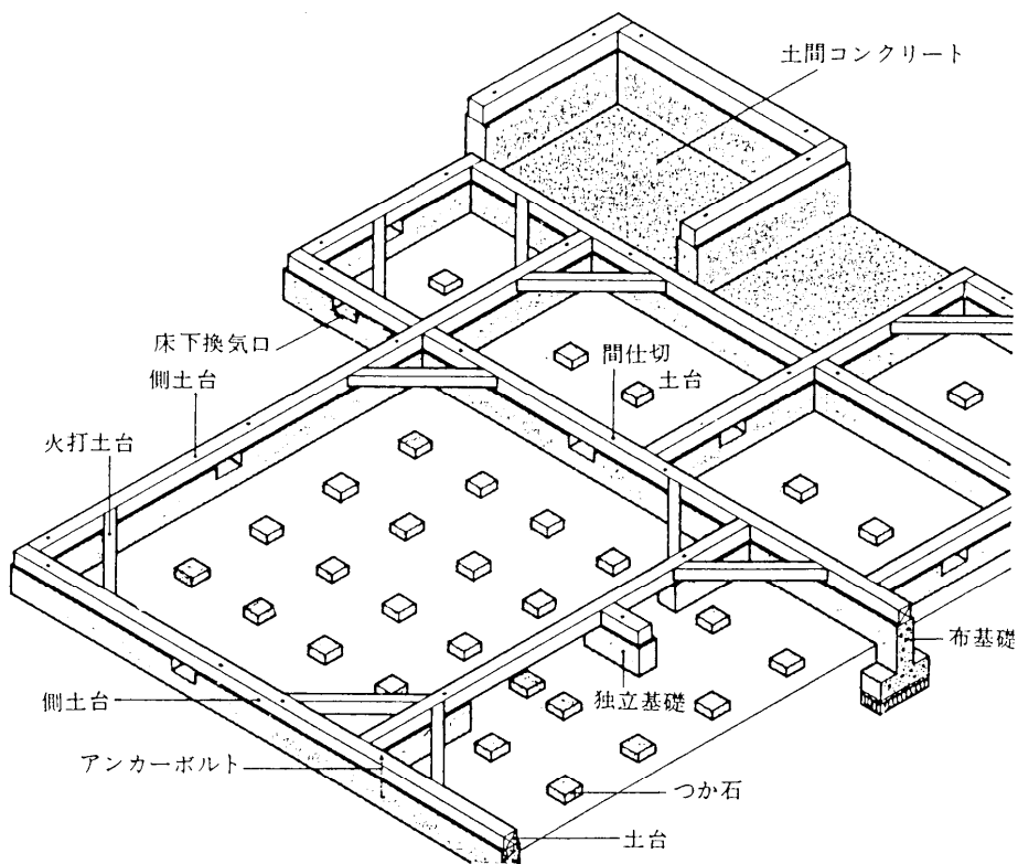
土台と基礎
