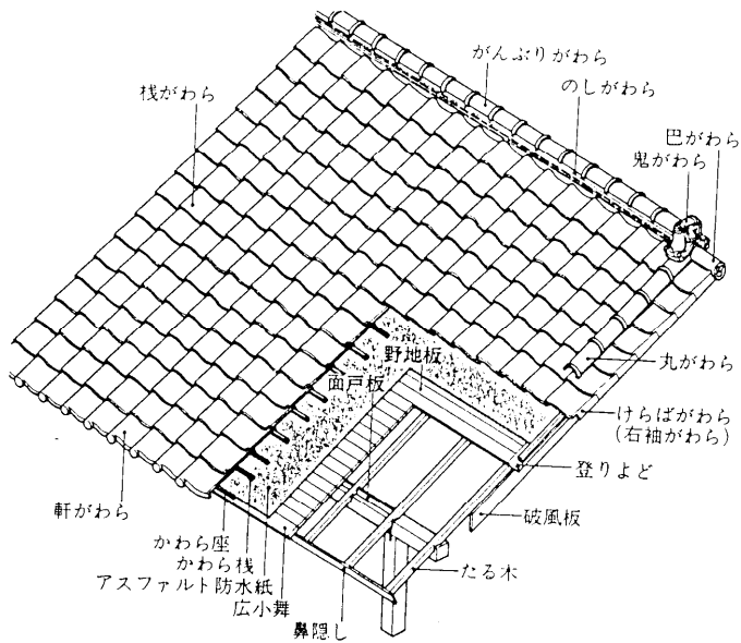
栈瓦葺き
