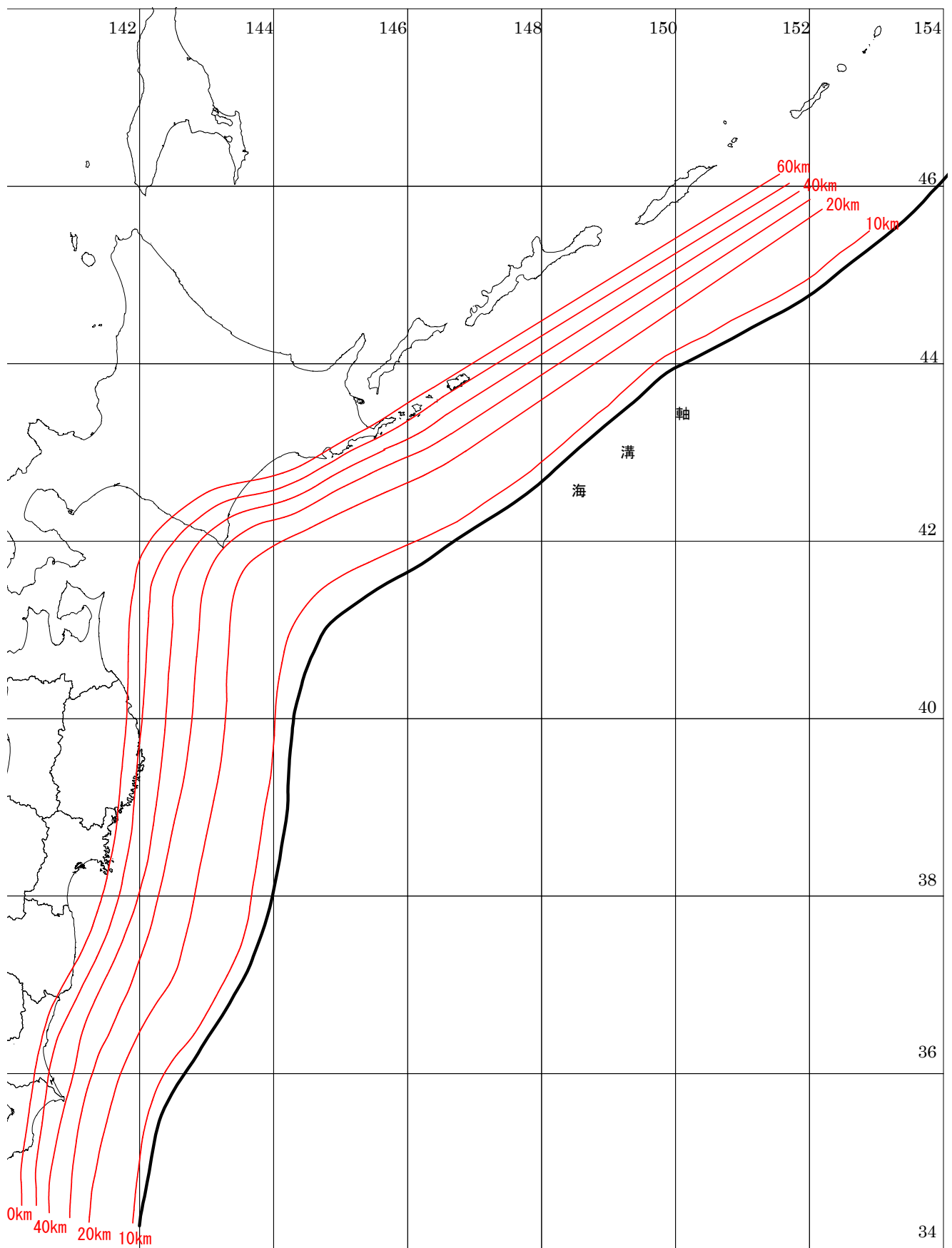
図 1 - 3 検討に用いるプレート形状
