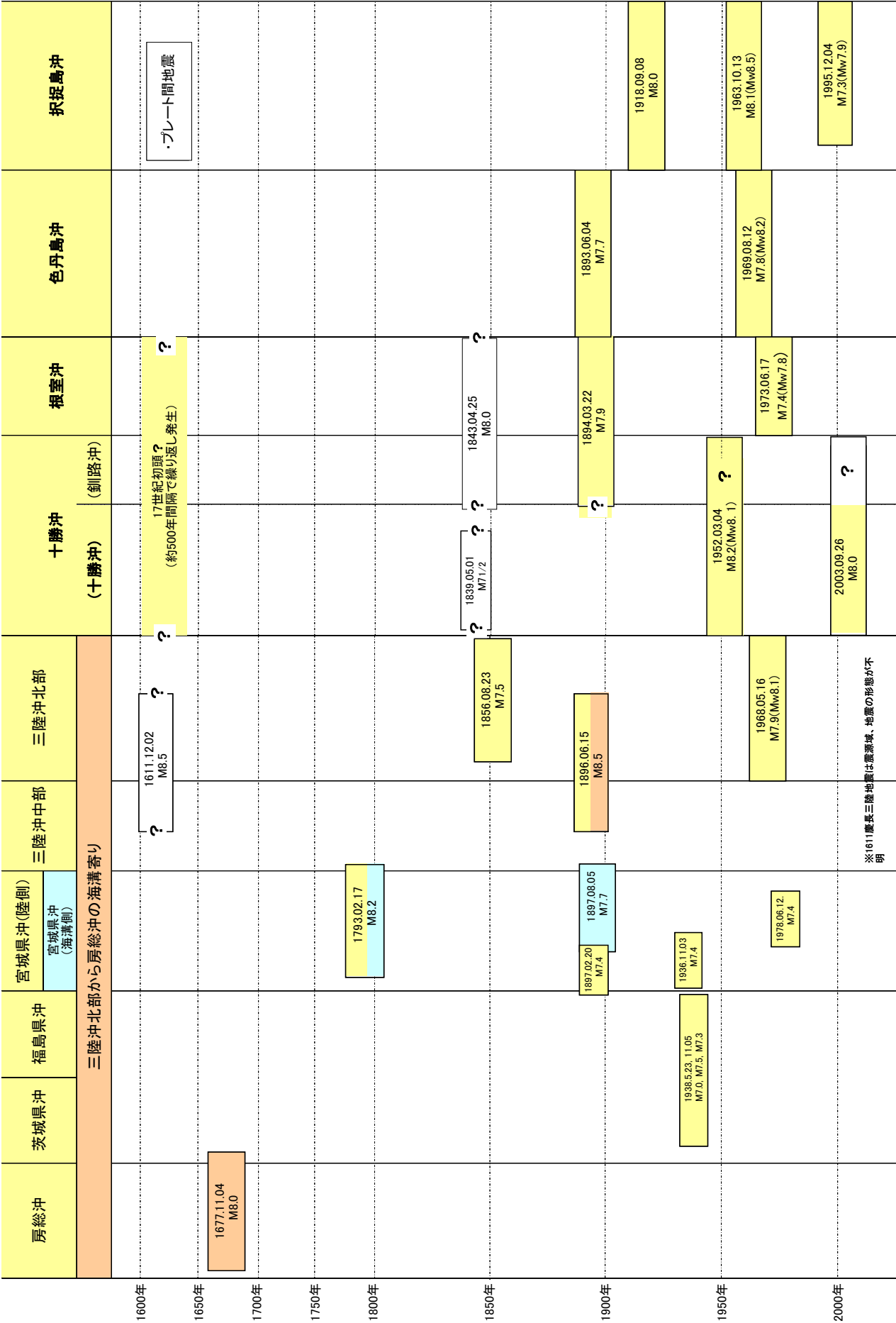
図1-2-2 日本海溝・千島海溝周辺の主なプレート間地震
