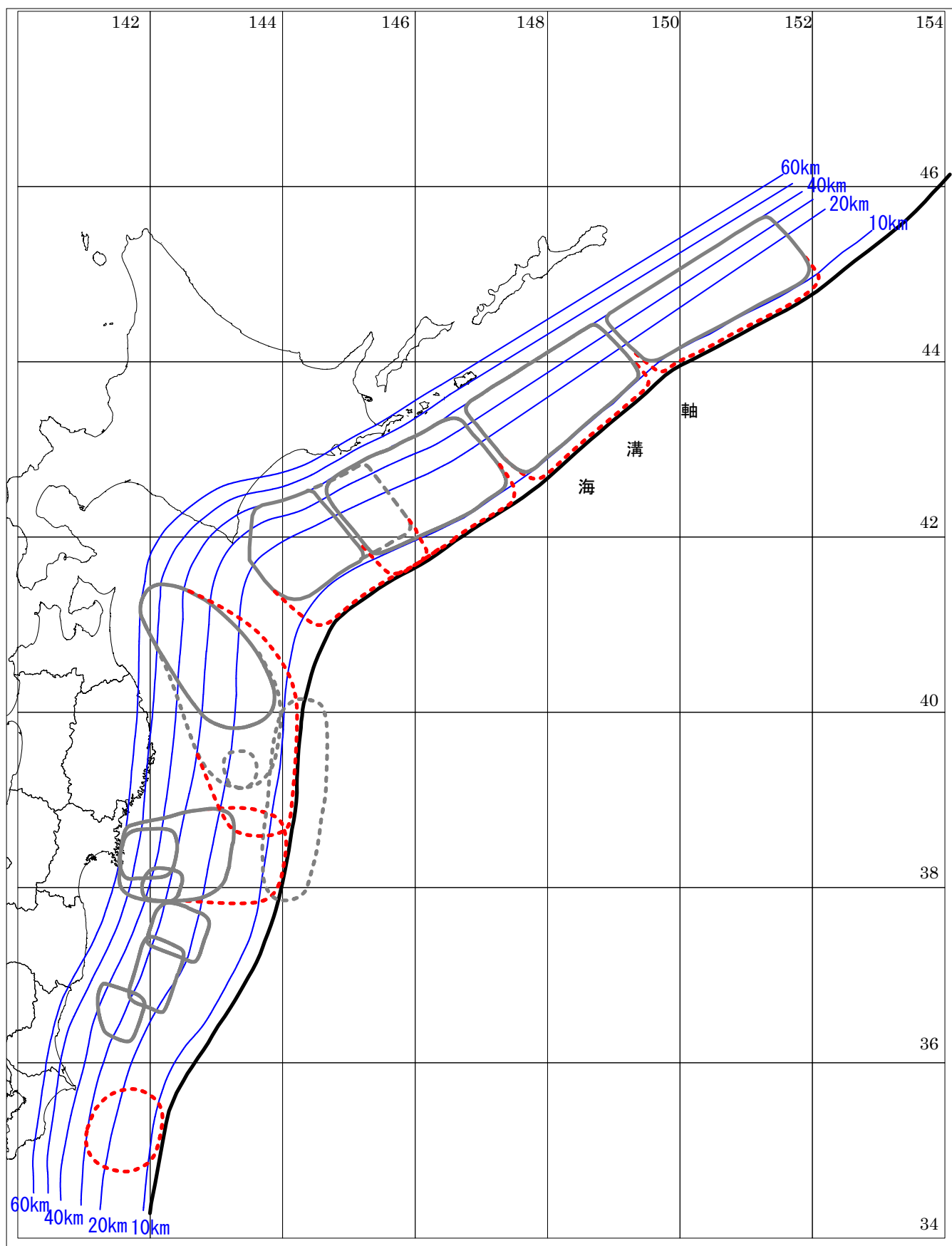
図 1 - 4 想定震源域
