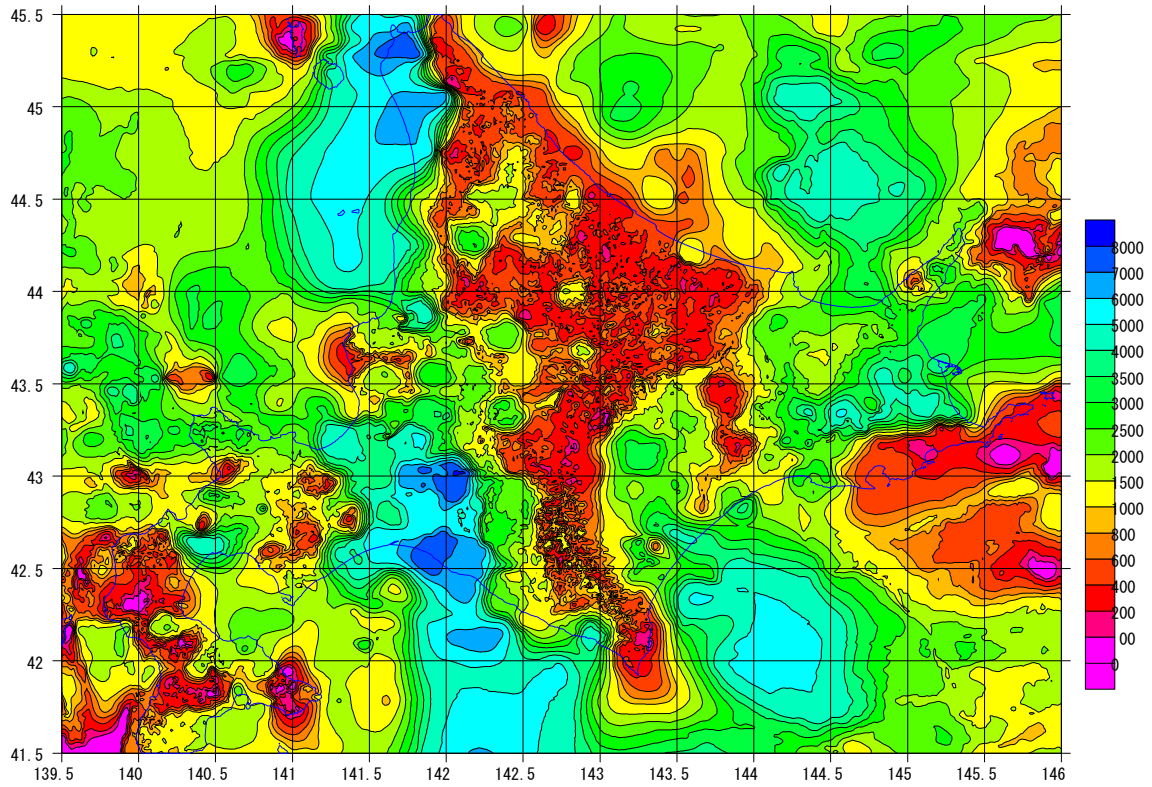
图 3-13 Vp4.7km/s 層(Vs2.4km/s 層)上面深度
