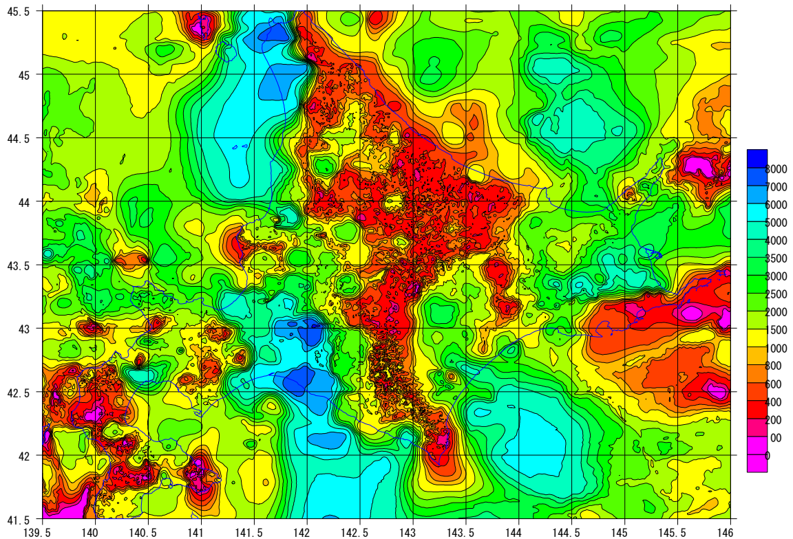
图 3-14 Vp5.5km/s 層上面深度(地震基盤 : Vs3.0km/s 層)
