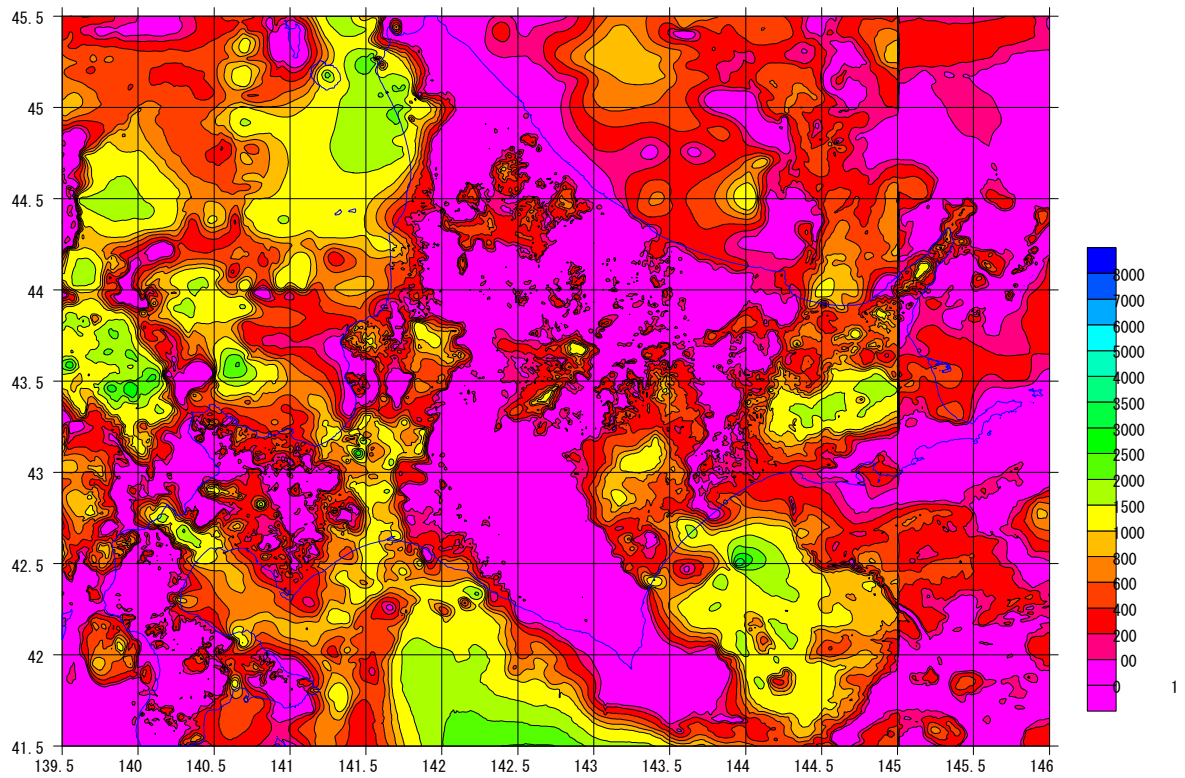
图 3-10 Vp2.5km/s 層(Vs1.0km/s 層)上面深度
