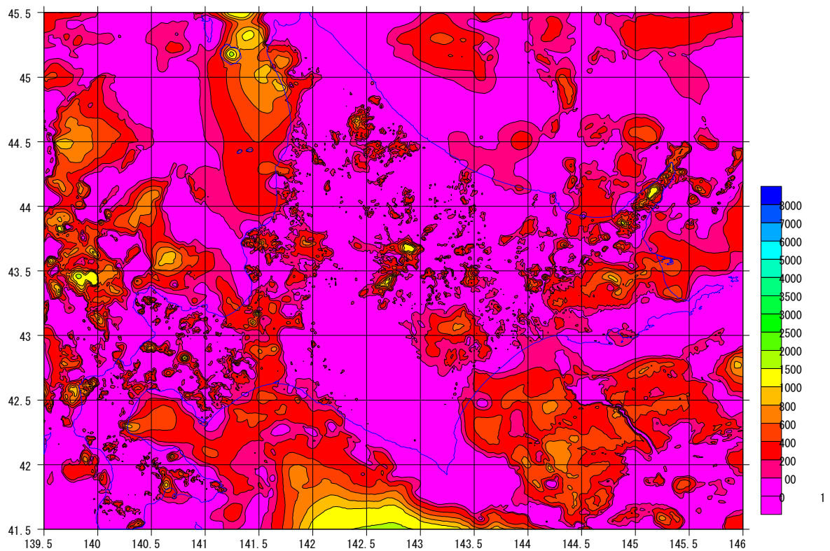
图 3-9 Vp2.1km/s 層上面深度(工学的基盤 : Vs0.7km/s 層)
