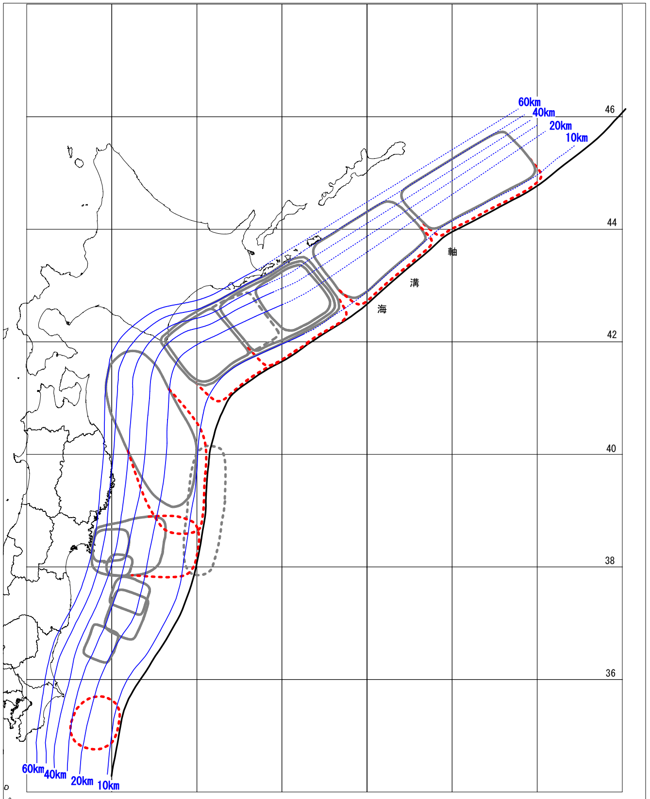
図 8 想定震源域
