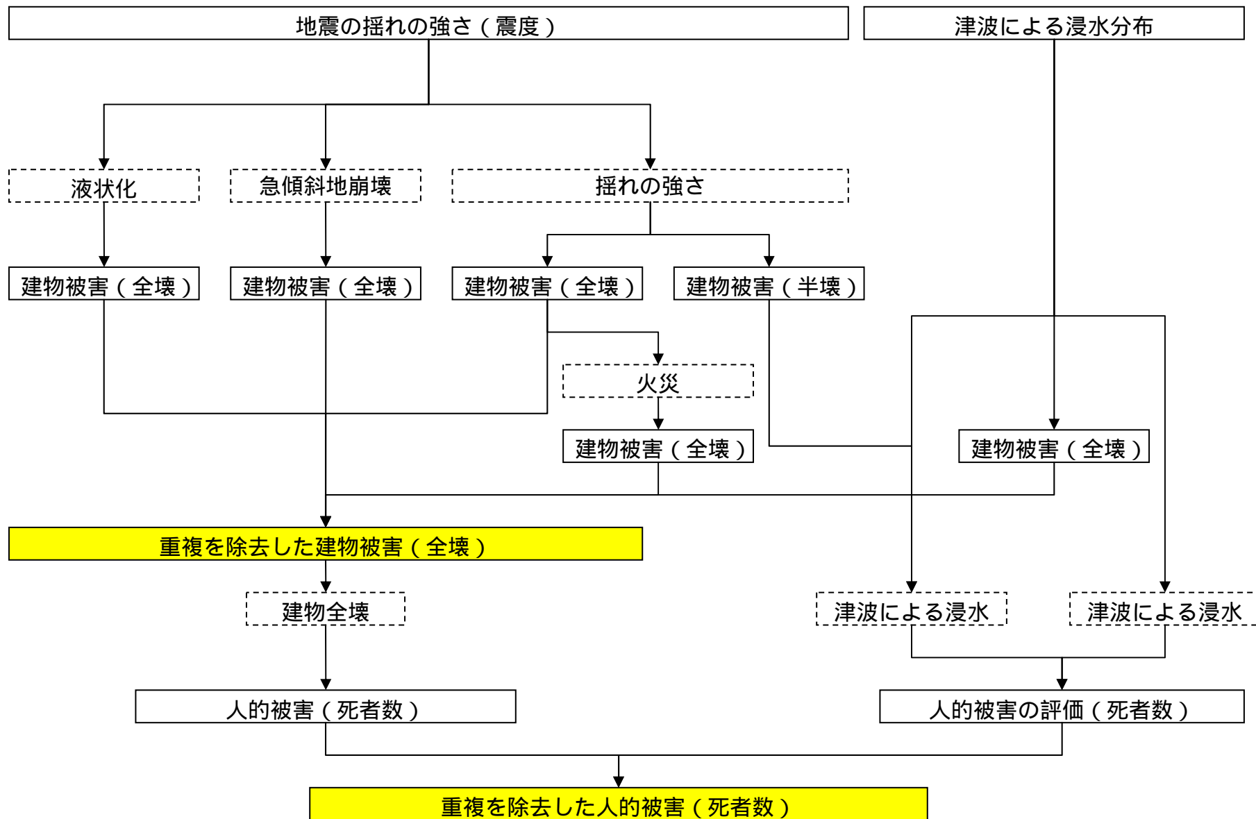
図 2 . 1 4 被害想定（人的・建物）のフローチャート
