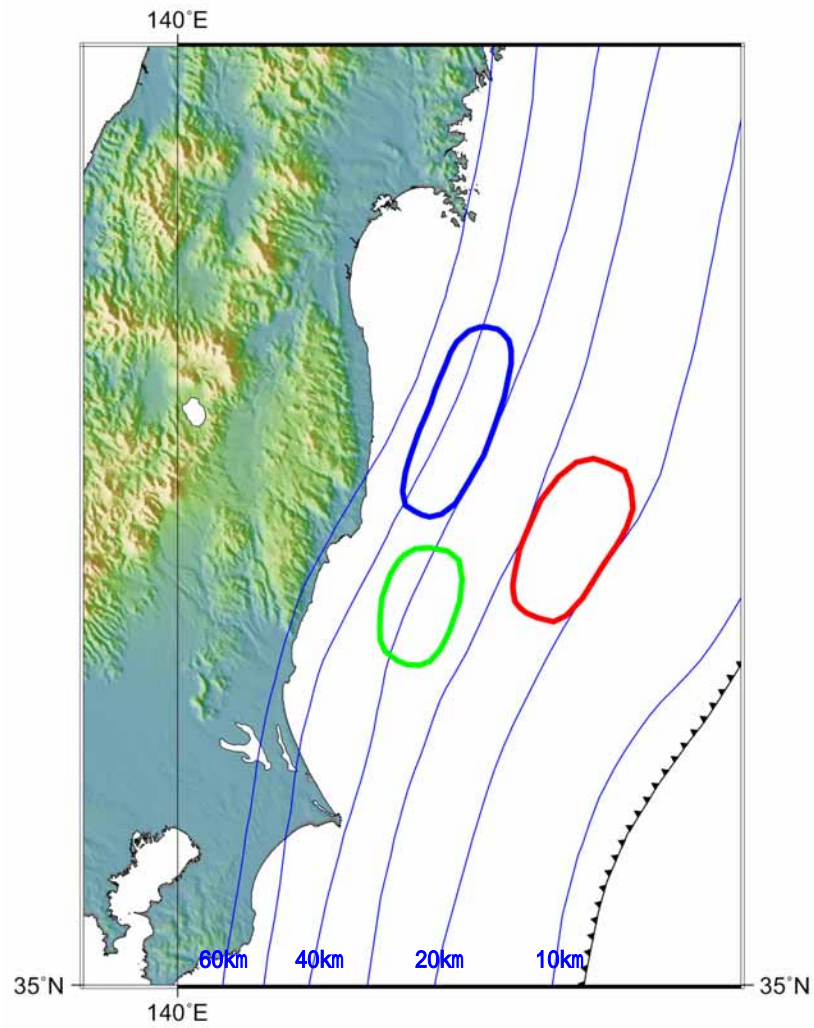
図 3-3-9-3 福島県沖の地震の断層モデル .
