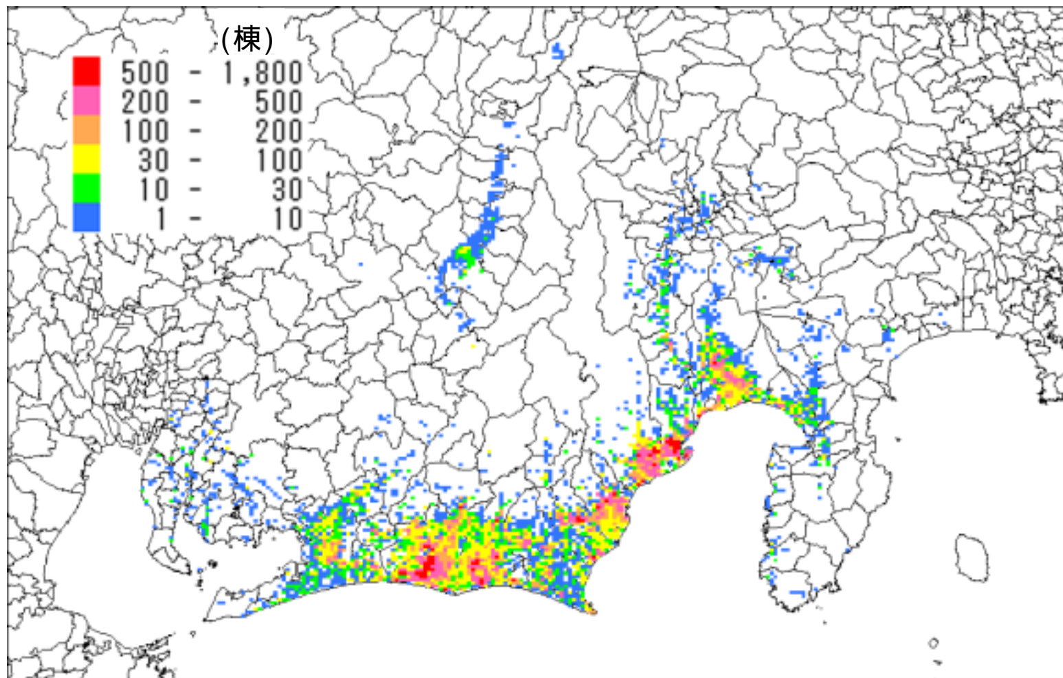
図3 最大ケースにおける地震の揺れによる建物被害の分布
