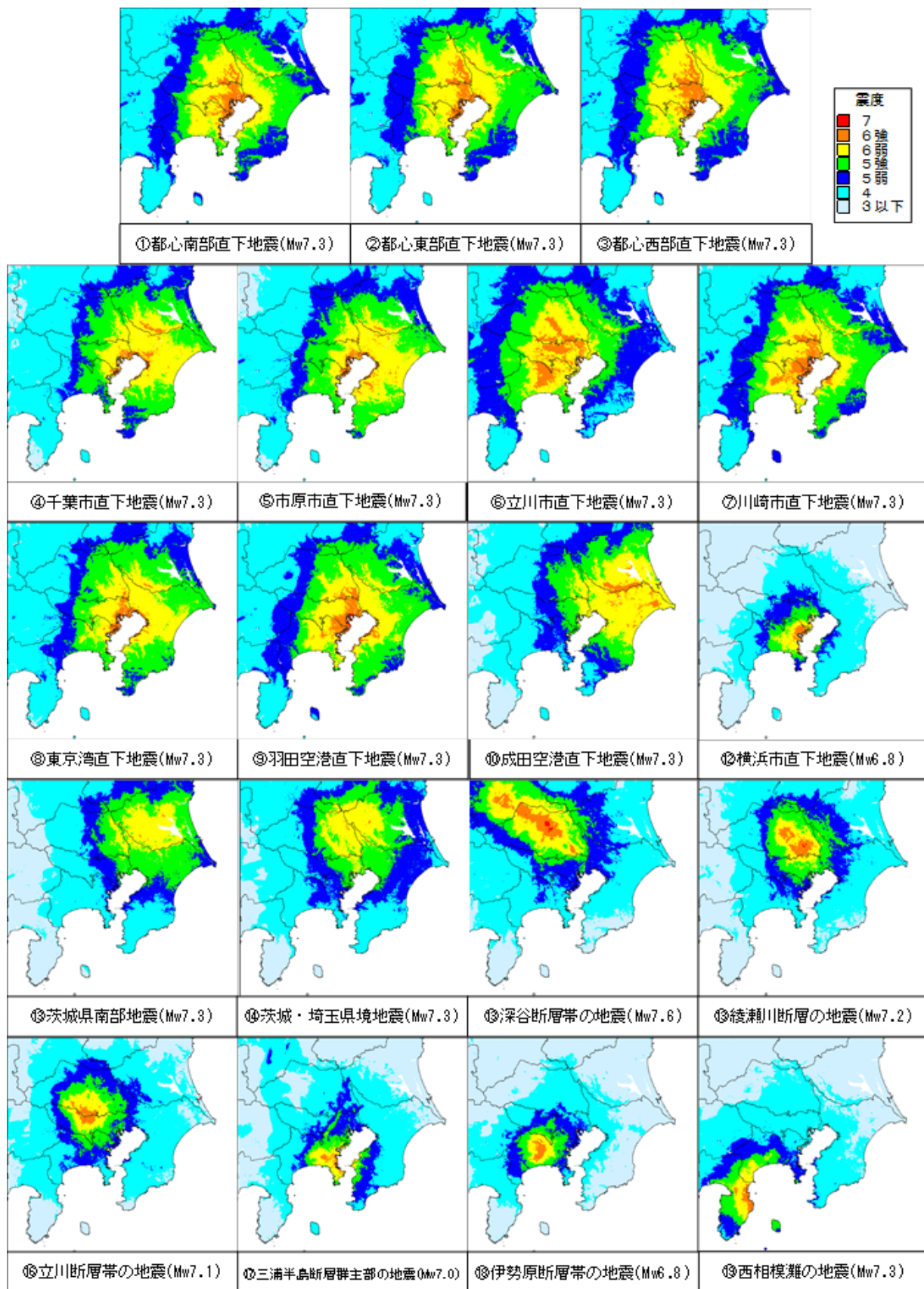
図1 首都直下のM7クラスの地震の震度分布(19地震) (「首都直下地震の被害想定と対策について(報告書)(令和7年12月公表)」より)
