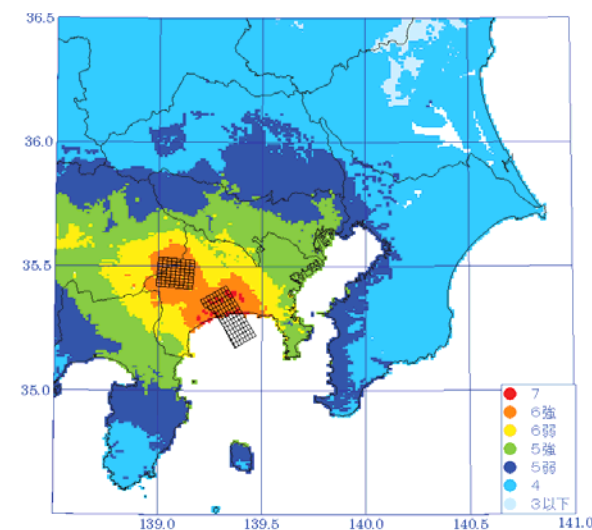
神縄・国府津一松田断層帯地震、M7.5
