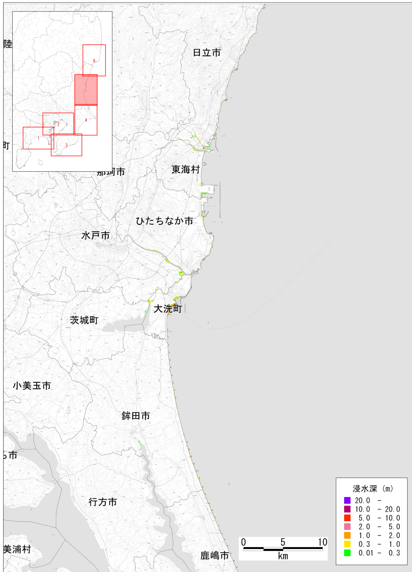
図 津波の浸水分布 【房総半島南東沖で想定されるタイプの地震】
