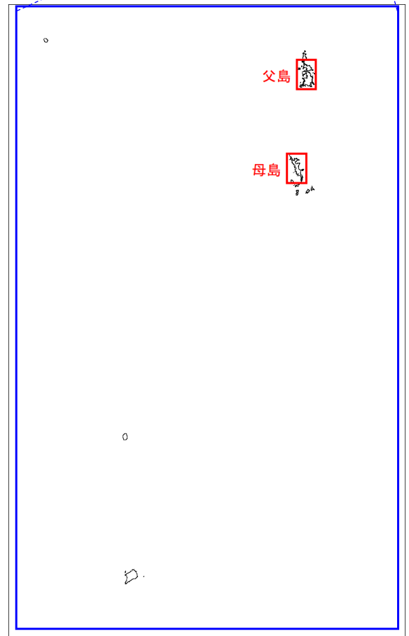
図 津波の浸水分布 【房総半島南東沖で想定されるタイプの地震】
