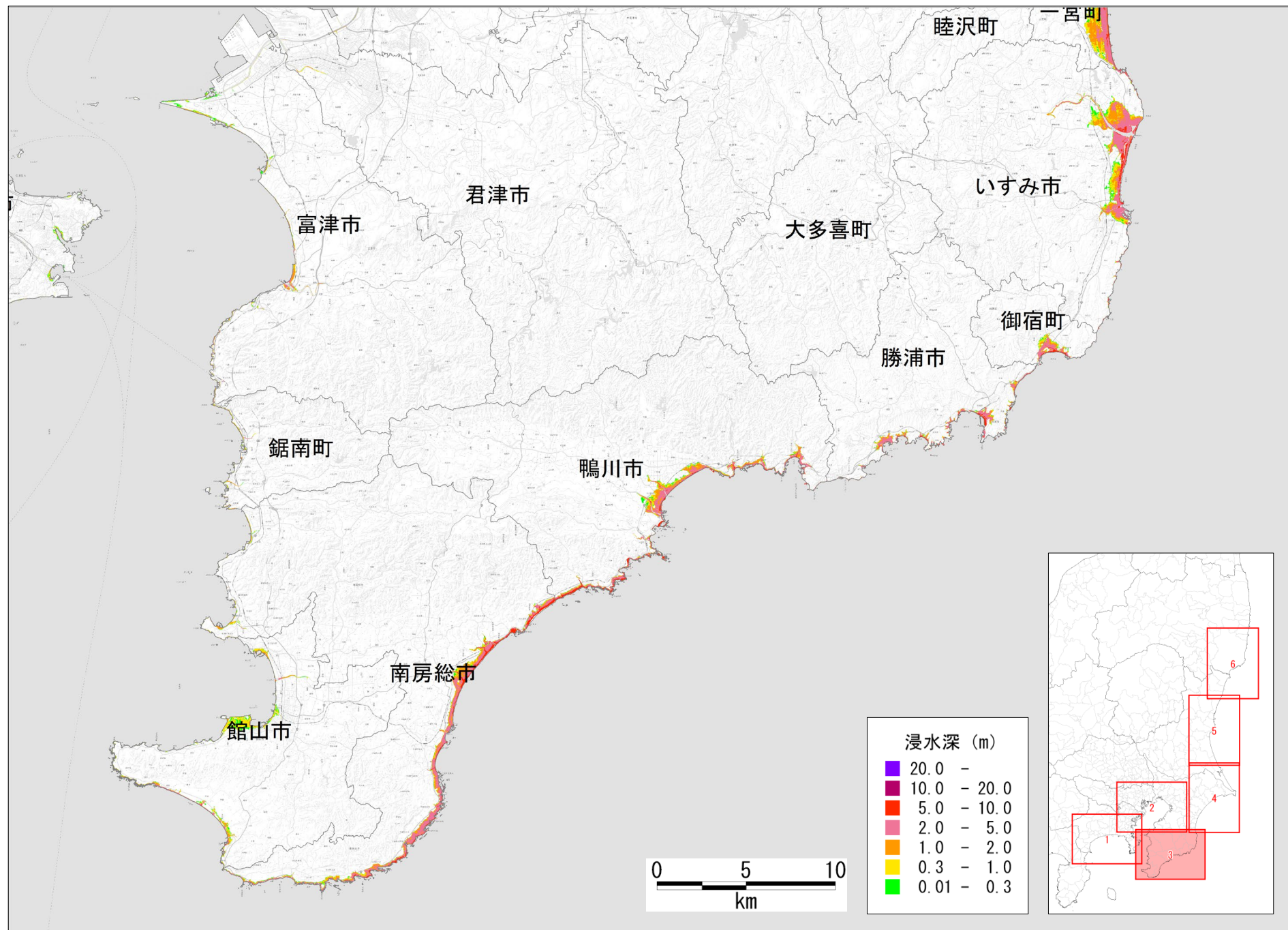
図 津波の浸水分布 【房総半島南東沖で想定されるタイプの地震】
