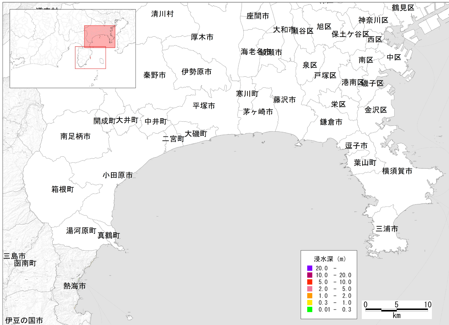
図 津波の浸水分布 【房総半島南東沖で想定されるタイプの地震】
