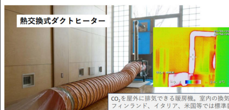
▲ダクトヒーターの使用状況（室内設置）
