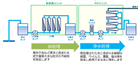
▲浄水施設の仕組み
