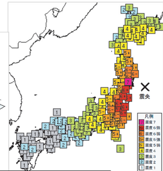
東北地方太平洋沖地震の津波高と震度分布
