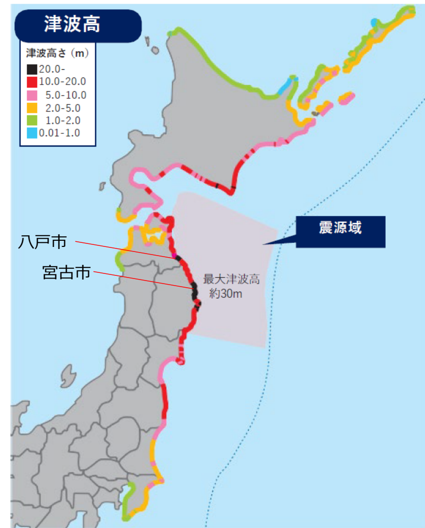
日本海溝モデル
