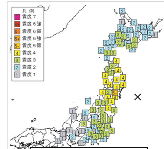
3/9地震の震源と震度分布
