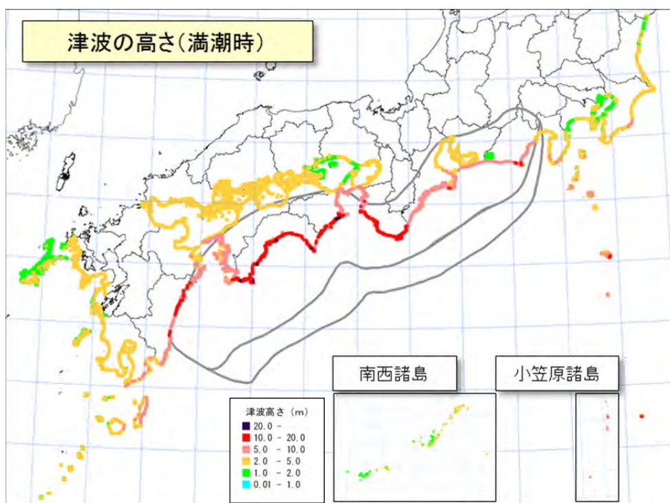
図5 津波高分布図（ケース3）
