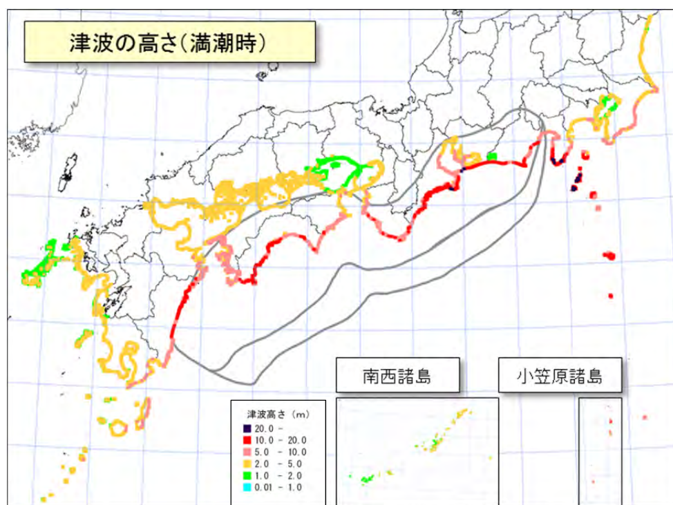
図4 津波高分布図（ケース1）
