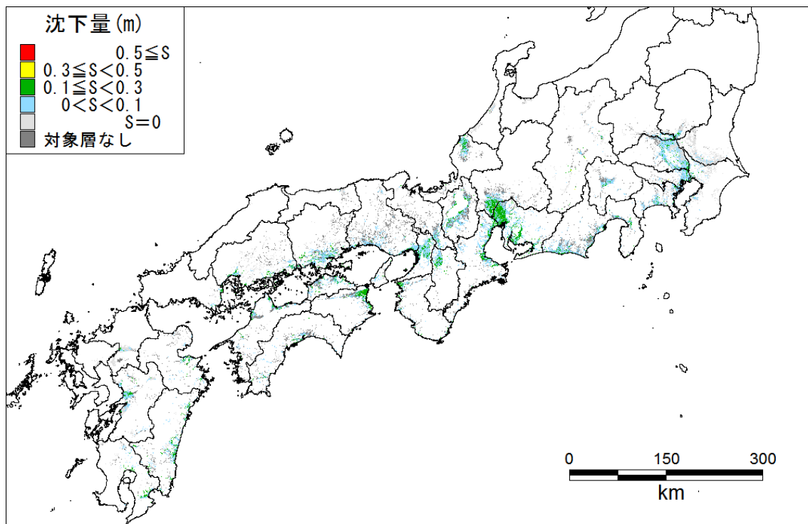
東側ケース 沈下量_全域
