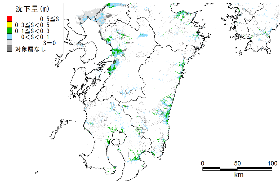
陸側ケース 沈下量_九州
