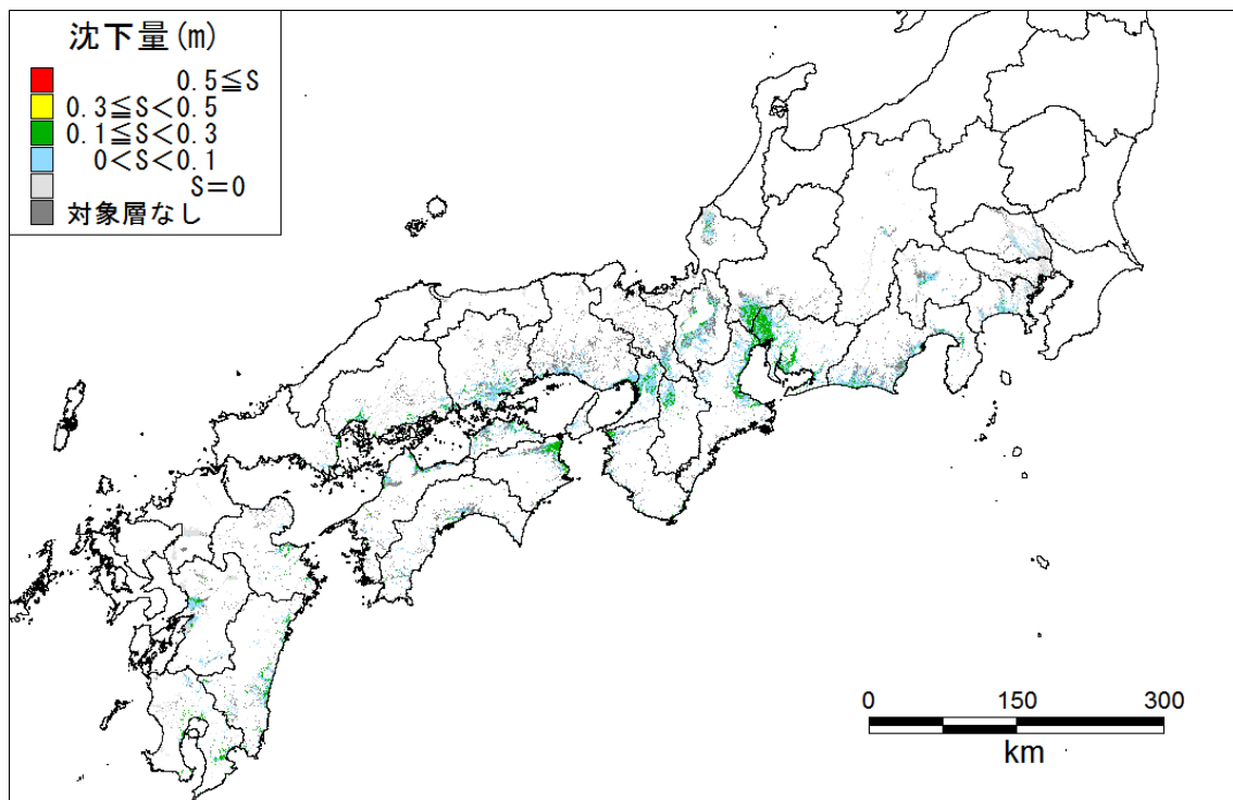
西側ケース 沈下量_全域
