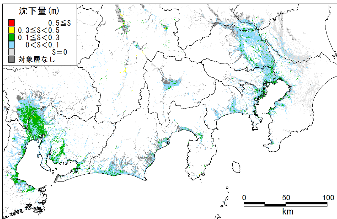
経験式 沈下量_関東-中部
