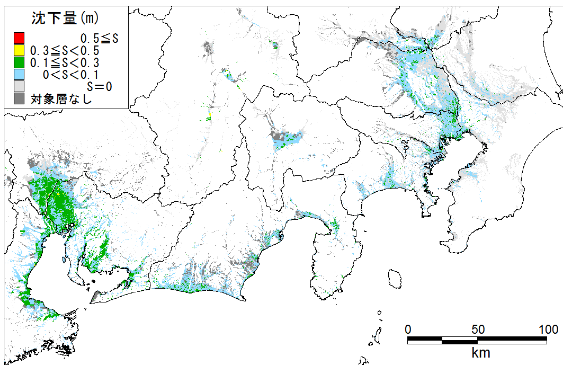
東側ケース 沈下量_関東-中部
