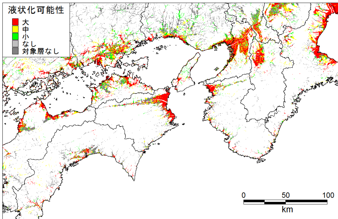
陸側ケース 液状化可能性_近畿-四国
