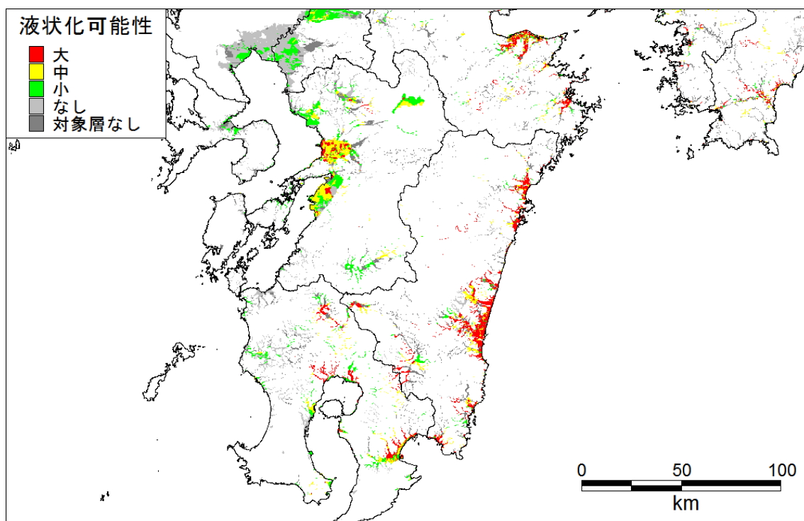
陸側ケース 液状化可能性_九州
