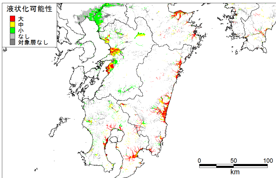
経験式 液状化可能性_九州
