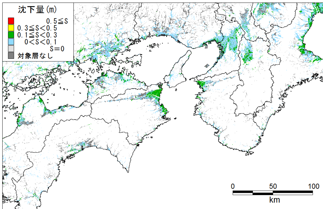
経験式 沈下量_近畿-四国
