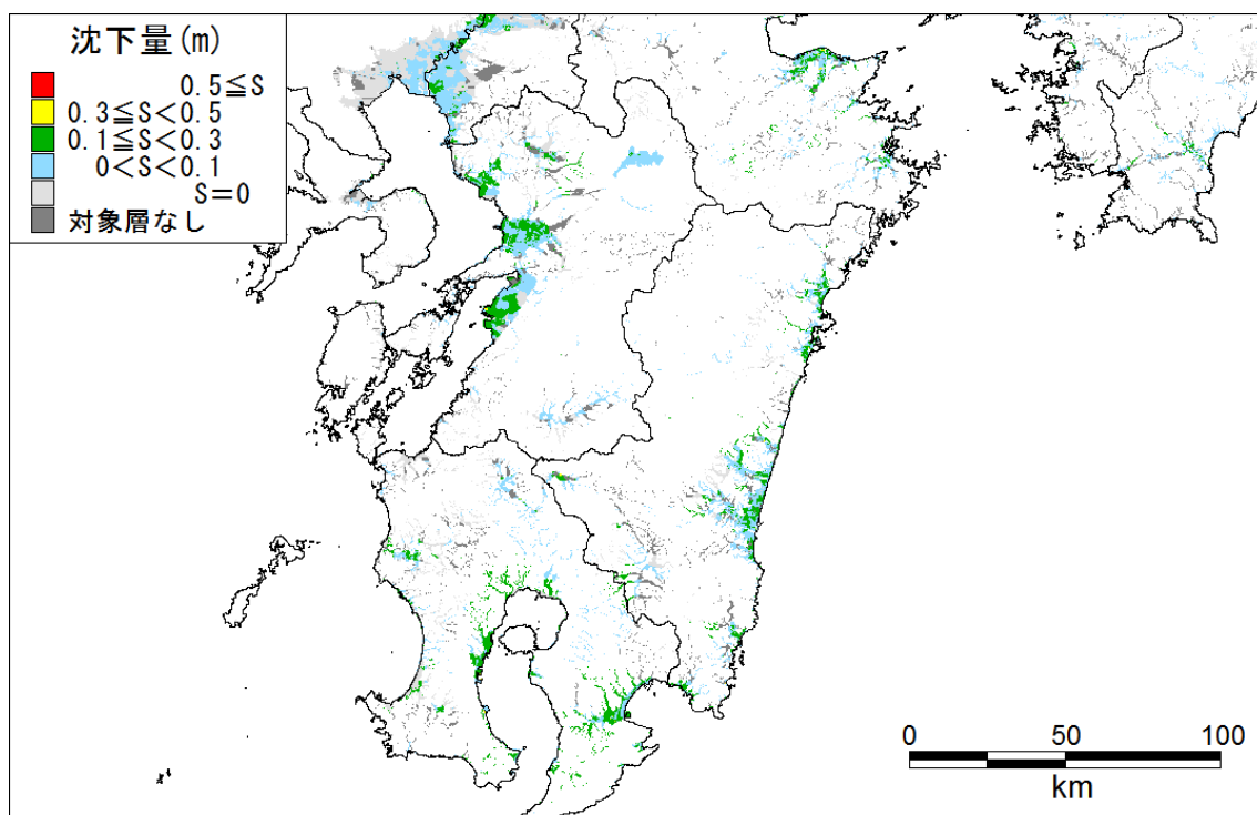
経験式 沈下量_九州
