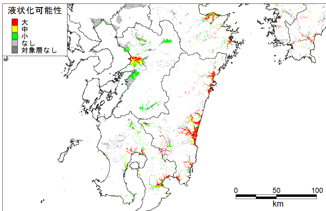
基本ケース 液状化可能性_九州
