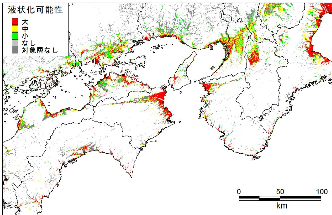
東側ケース 液状化可能性_近畿-四国
