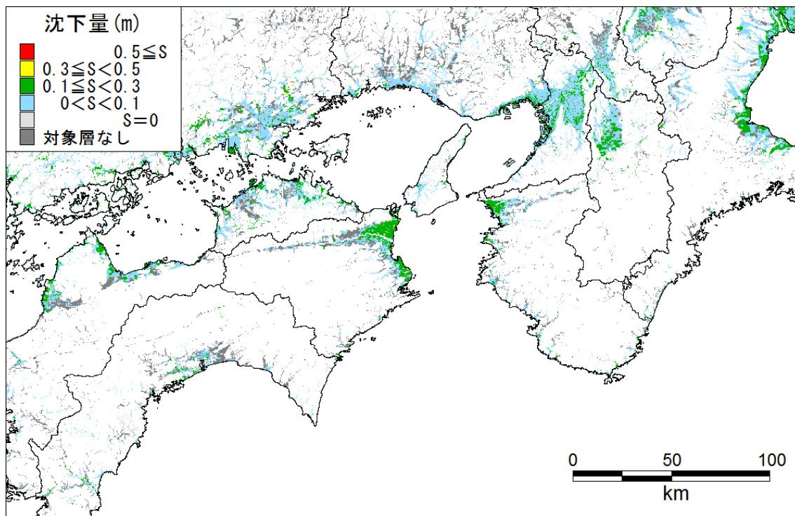
陸側ケース 沈下量_近畿-四国
