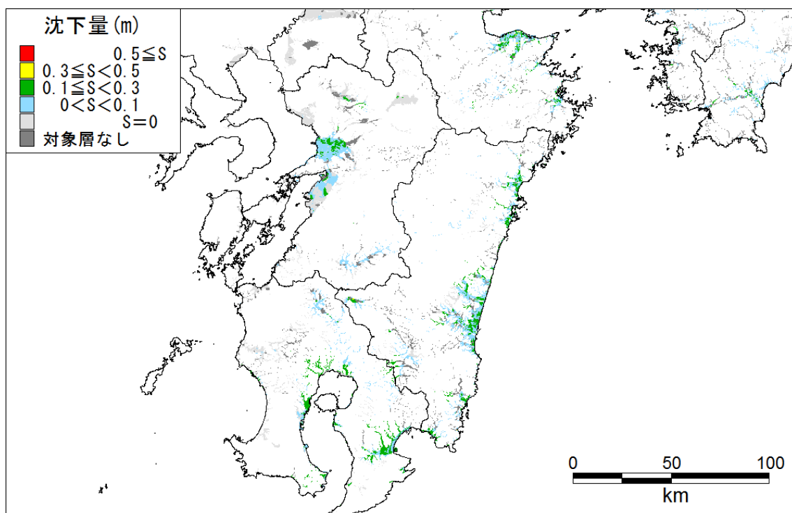
西側ケース 沈下量_九州
