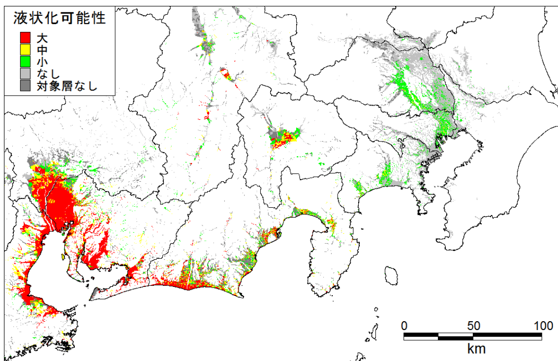
陸側ケース 液状化可能性_関東-中部
