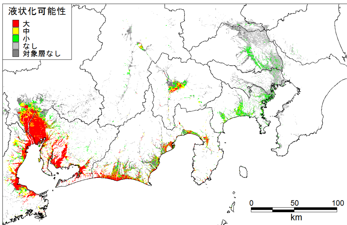
基本ケース 液状化可能性_関東-中部
