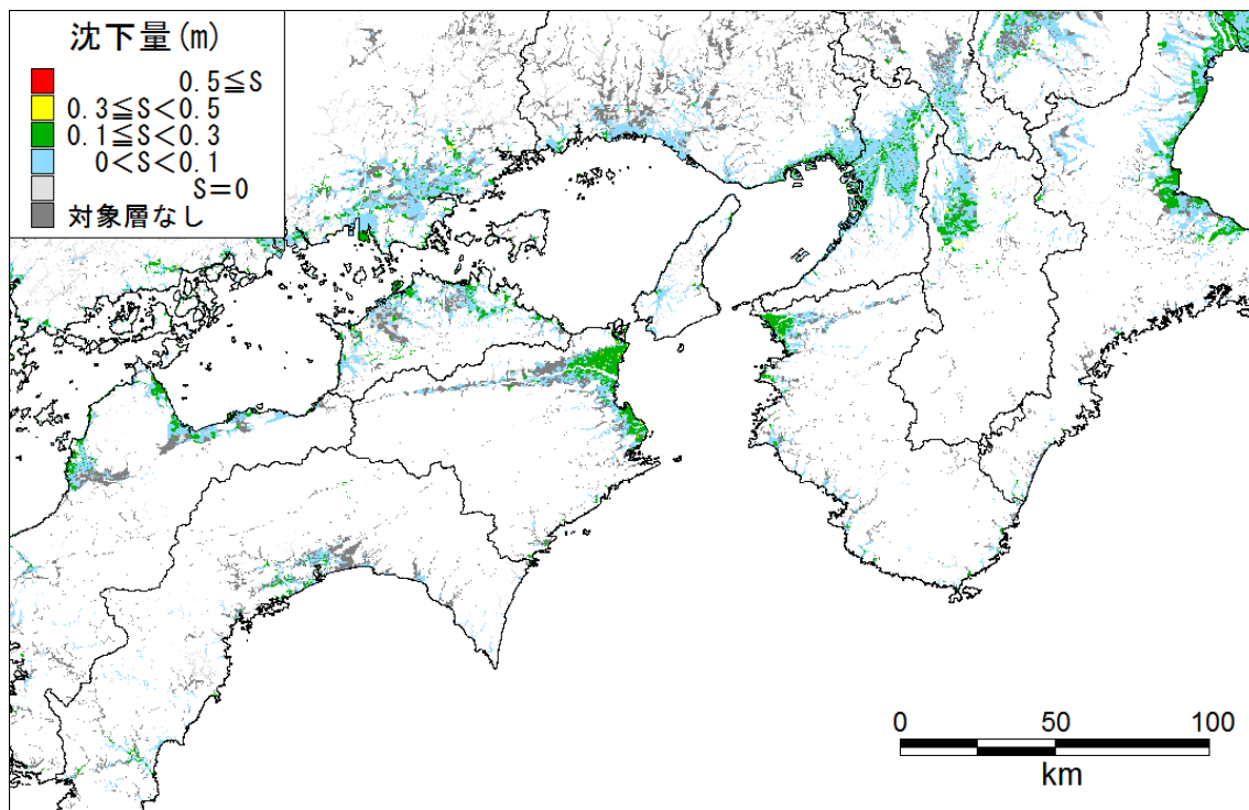
基本ケース 沈下量_近畿-四国
