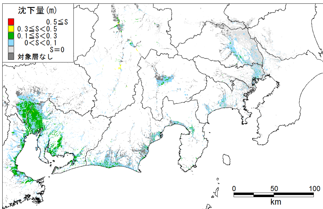
陸側ケース 沈下量_関東-中部
