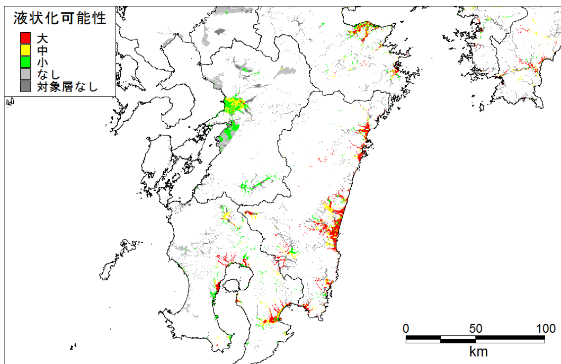
西側ケース 液状化可能性_九州
