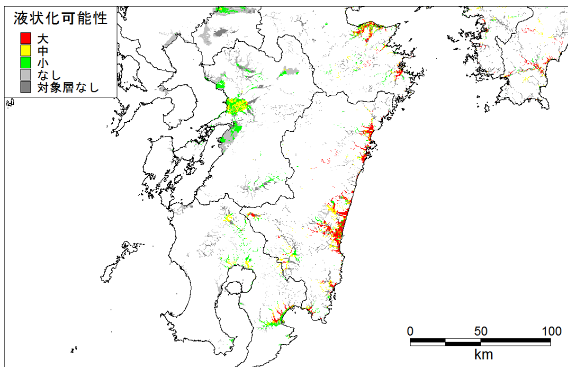
東側ケース 液状化可能性_九州
