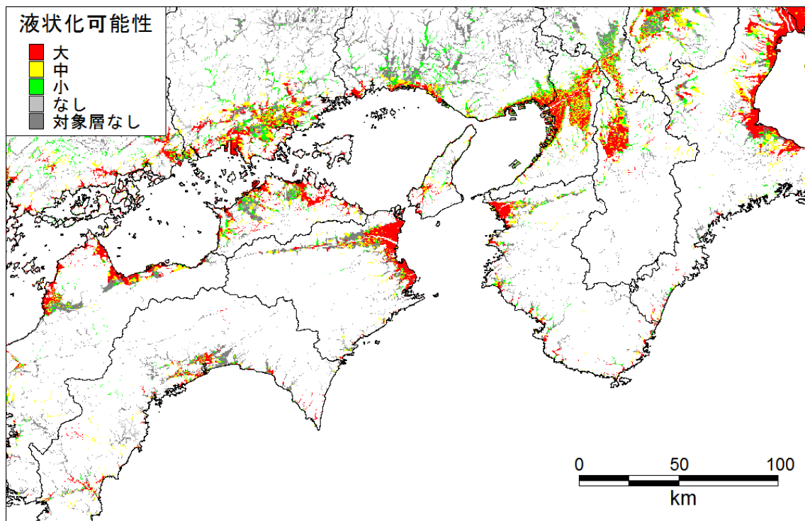
経験式 液状化可能性_近畿-四国
