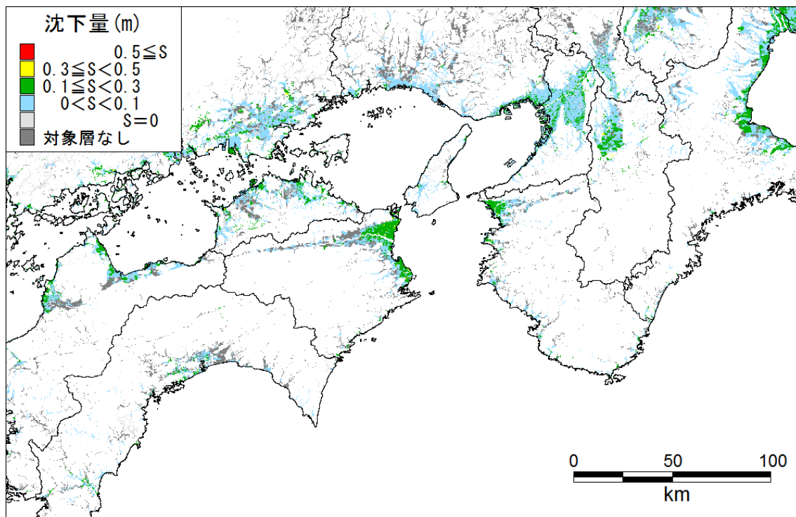
東側ケース 沈下量_近畿-四国
