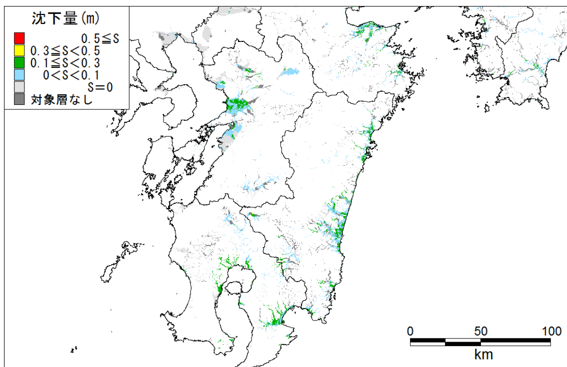
基本ケース 沈下量_九州
