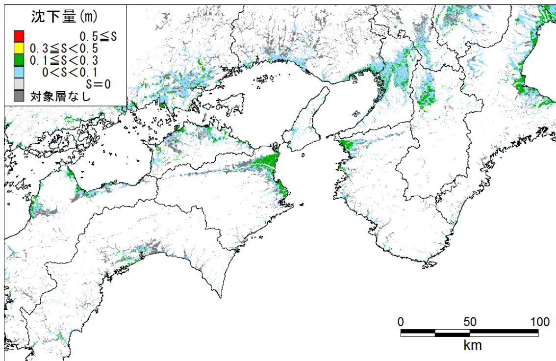
西側ケース 沈下量_近畿-四国
