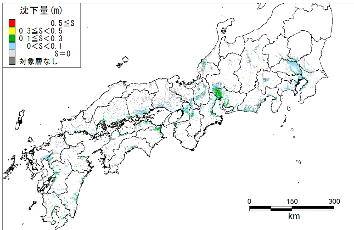
経験式 沈下量_全域
