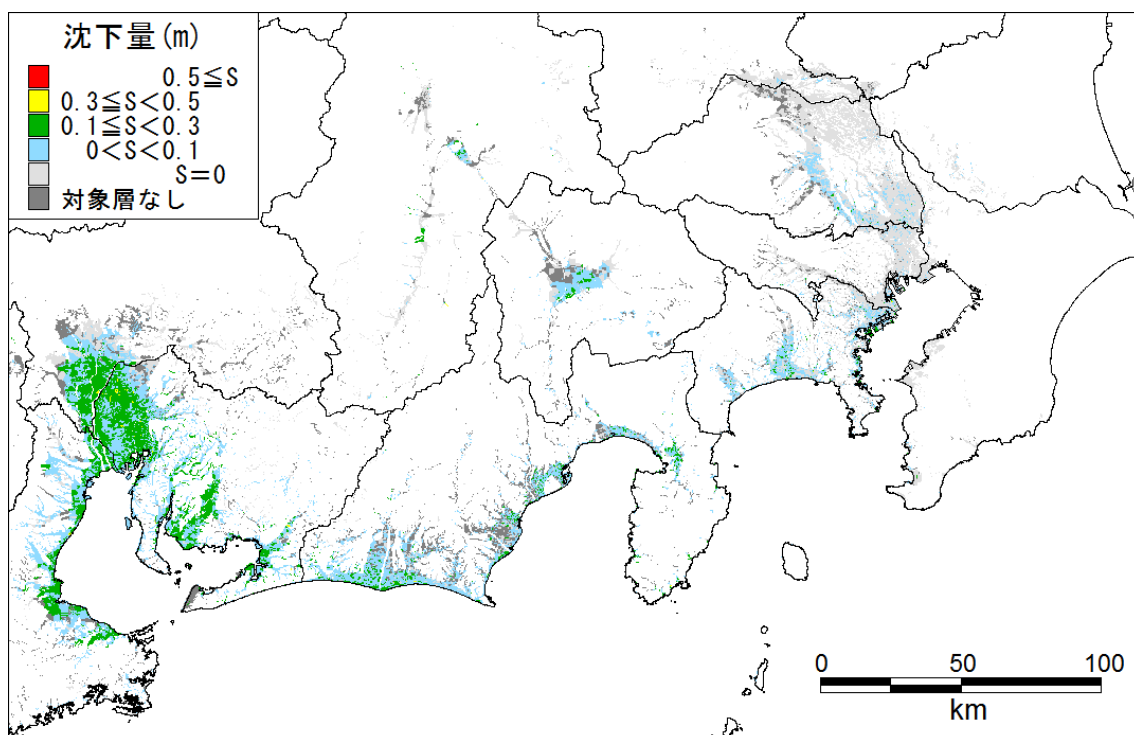
基本ケース 沈下量_関東-中部
