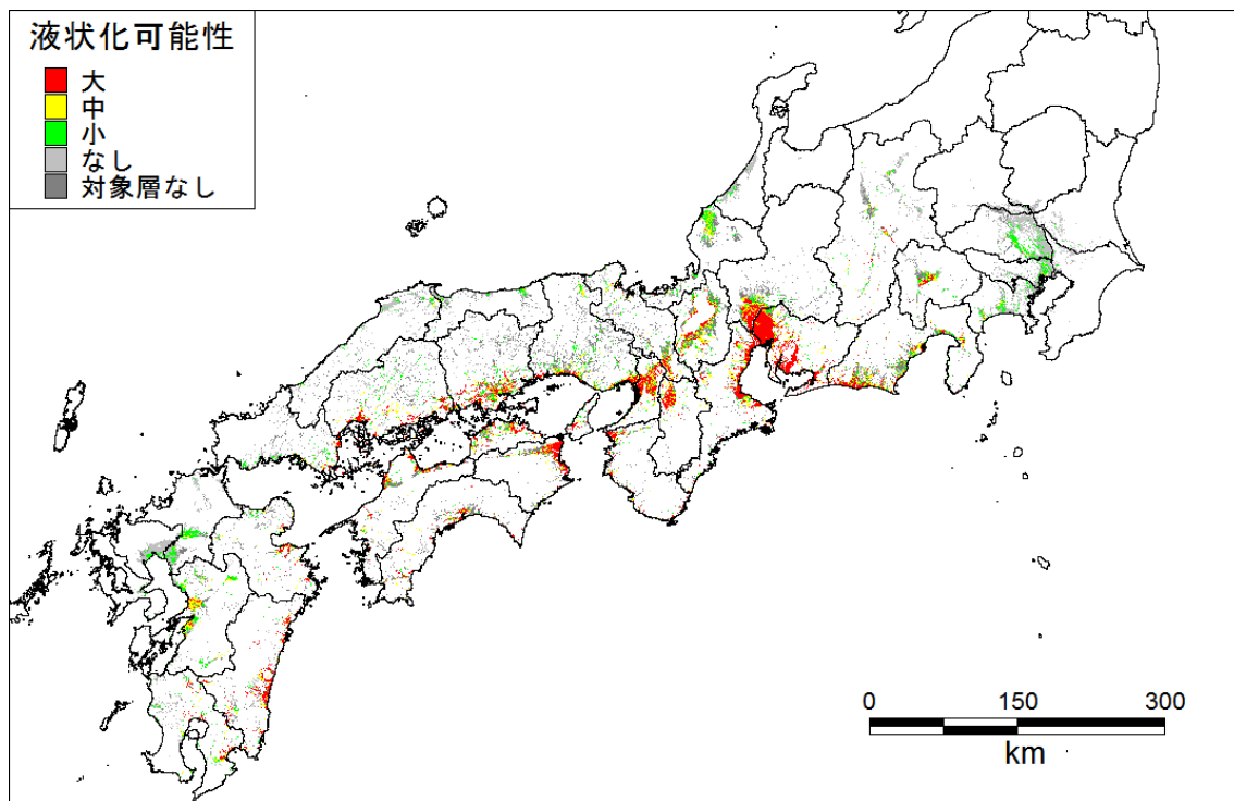
陸側ケース 液状化可能性_全域
