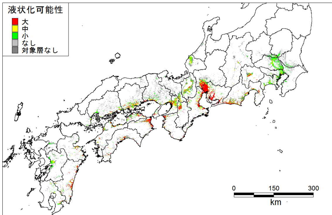
東側ケース 液状化可能性_全域
