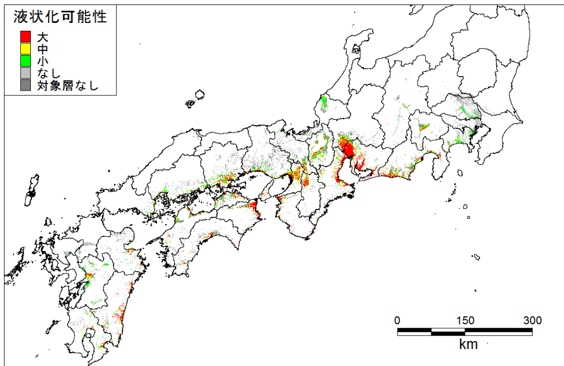
基本ケース 液状化可能性_全域
