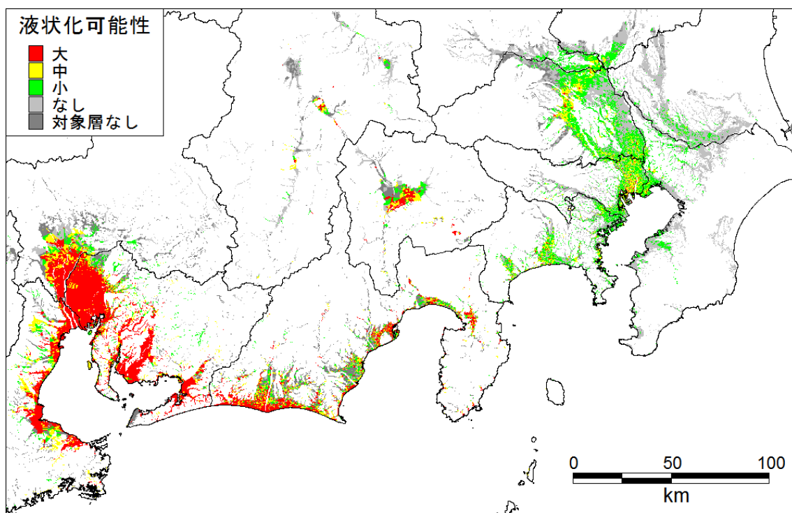
東側ケース 液状化可能性_関東-中部
