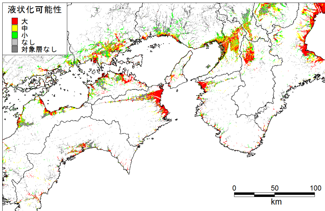
西側ケース 液状化可能性_近畿-四国
