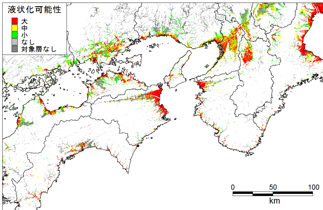
基本ケース 液状化可能性_近畿-四国
