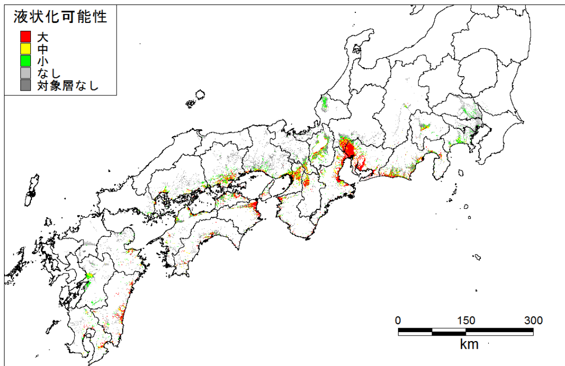
西側ケース 液状化可能性_全域
