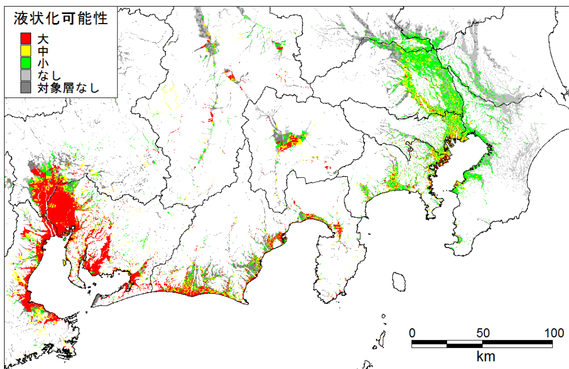
経験式 液状化可能性_関東-中部
