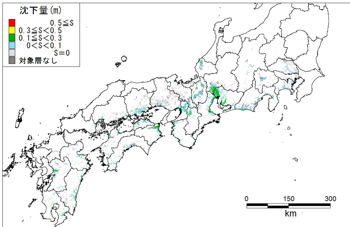
基本ケース 沈下量_全域
