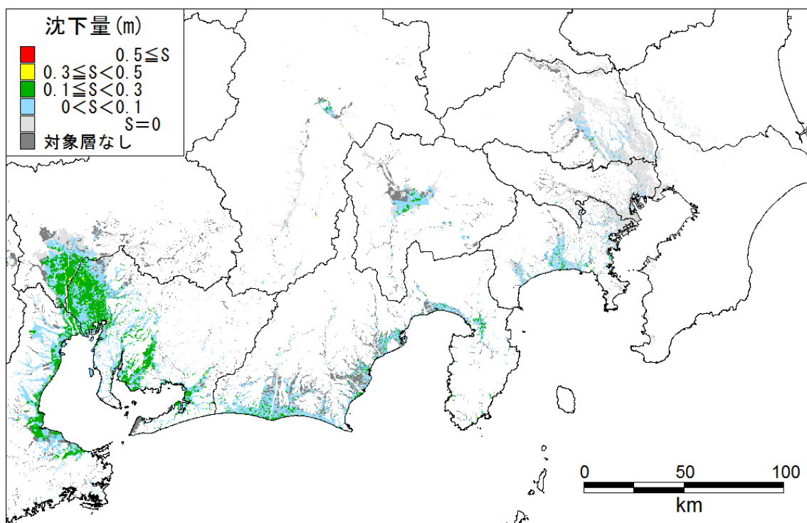
西側ケース 沈下量_関東-中部
