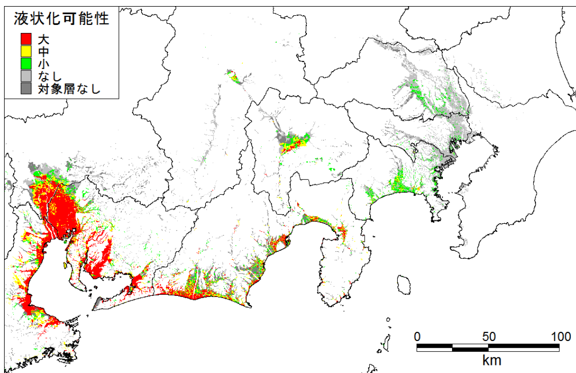
西側ケース 液状化可能性_関東-中部
