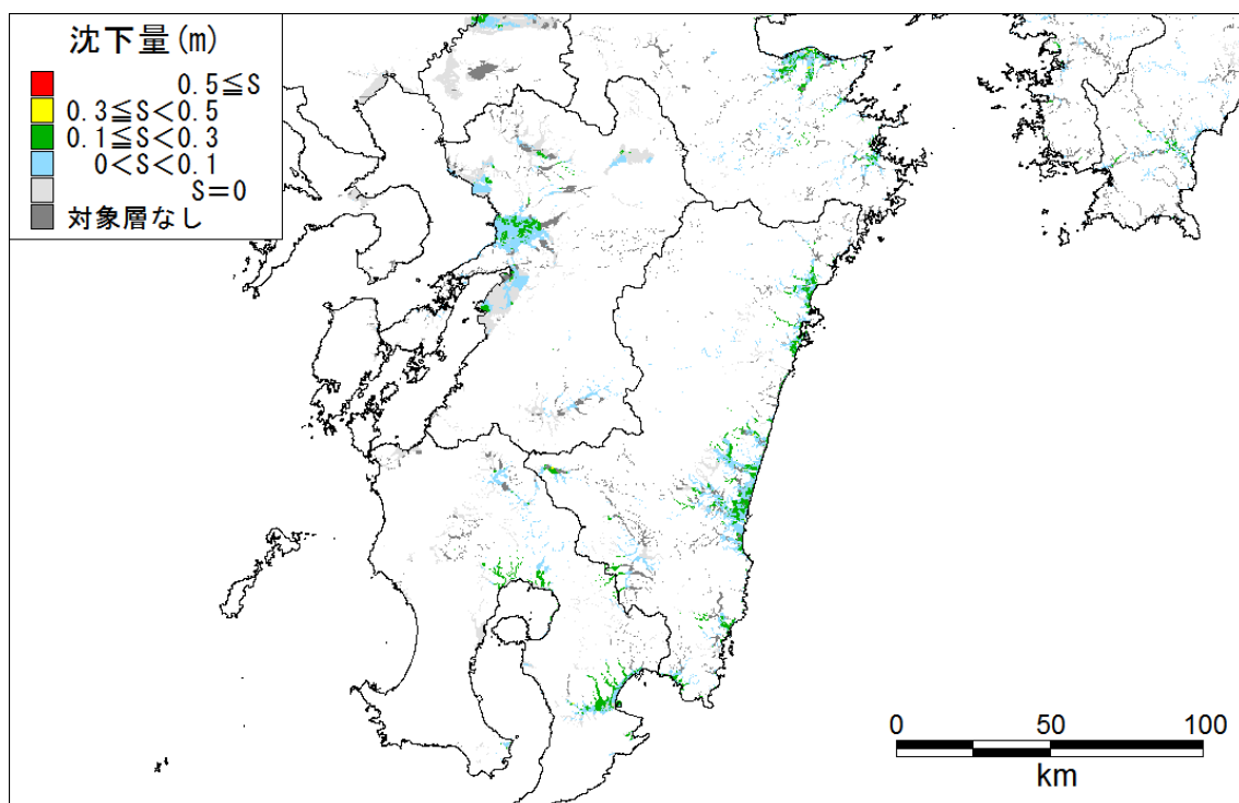
東側ケース 沈下量_九州
