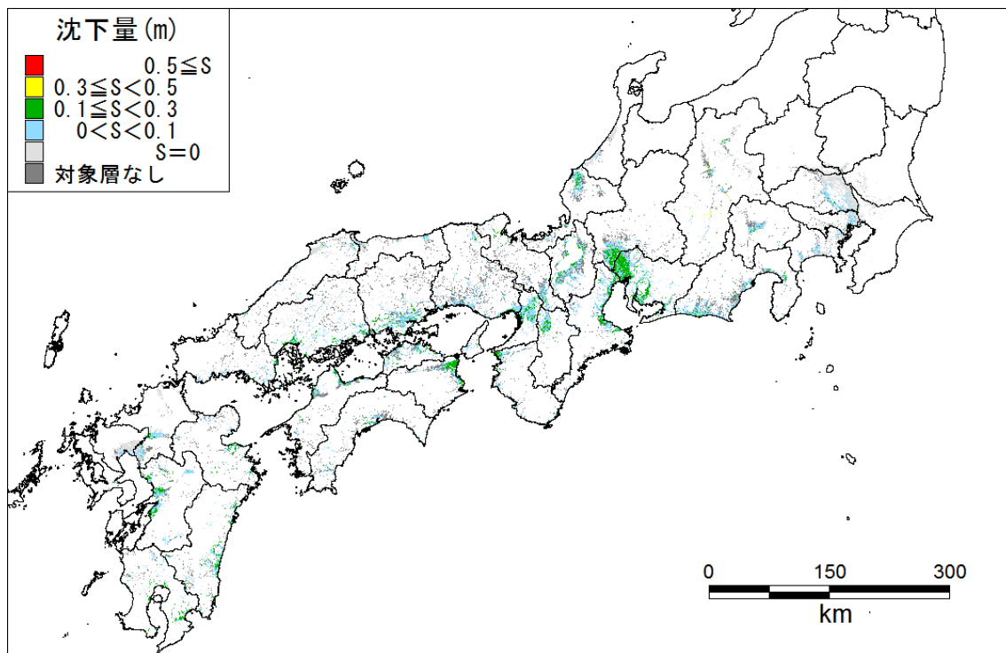
陸側ケース 沈下量_全域
