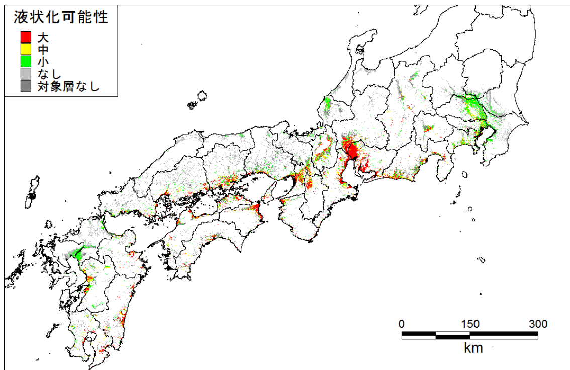
経験式 液状化可能性_全域
