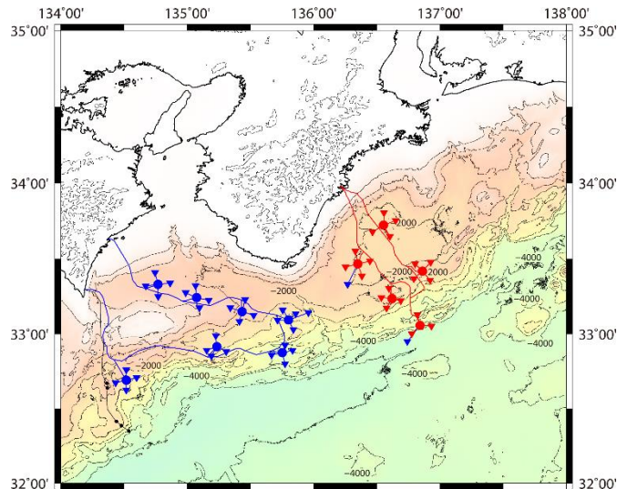
地震・津波監視システム(地震・水圧の観測) 【防災科学技術研究所】
