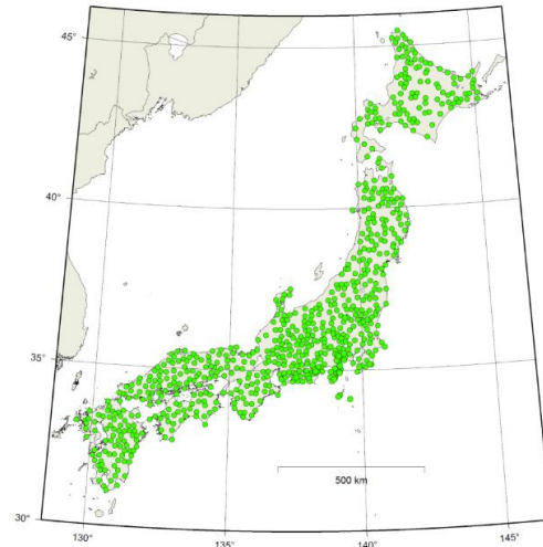
高感度地震観測網(地震・傾斜の観測) 【防災科学技術研究所】
