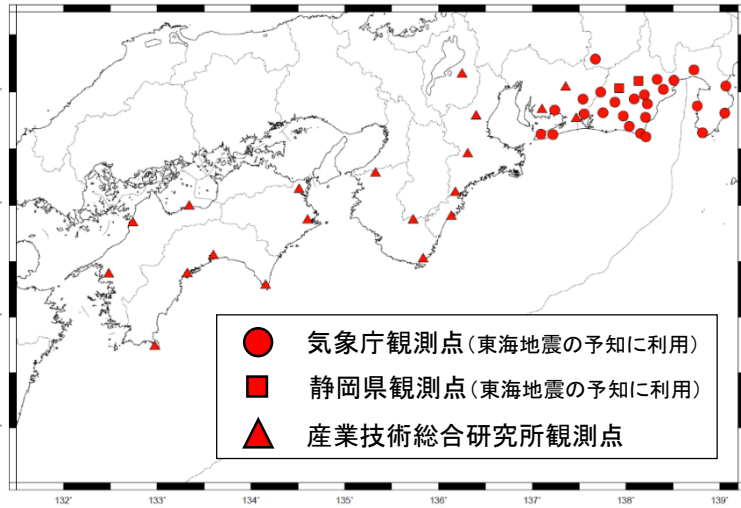
地殻のひずみ観測点【気象庁・静岡県】 地下水等総合観測点(地殻のひずみ・地下水位の観測) 【産業技術総合研究所】
