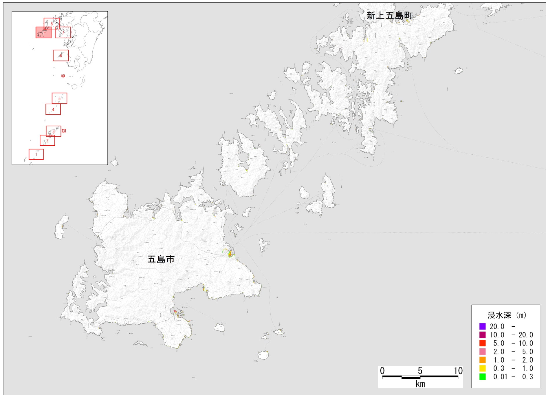
図 津波の浸水分布 【最大クラスケース③、堤防条件：津波が乗り越えたら破堤する】
