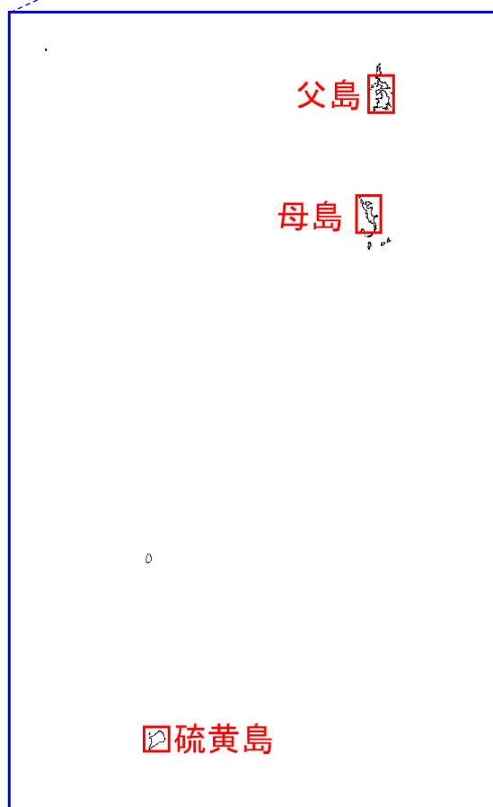
図 津波の浸水分布 【最大クラスケース③、堤防条件：津波が乗り越えたら破堤する】
