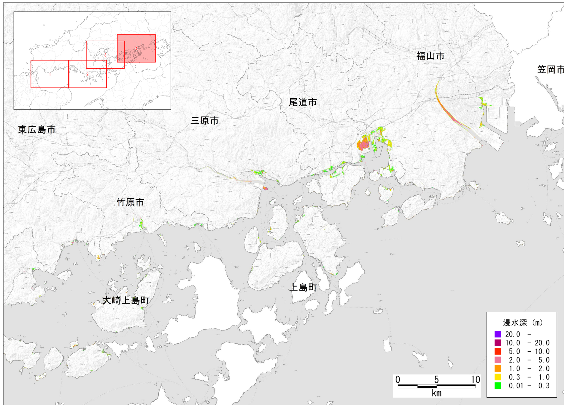
図 津波の浸水分布 【最大クラスケース③、堤防条件：津波が乗り越えたら破堤する】
