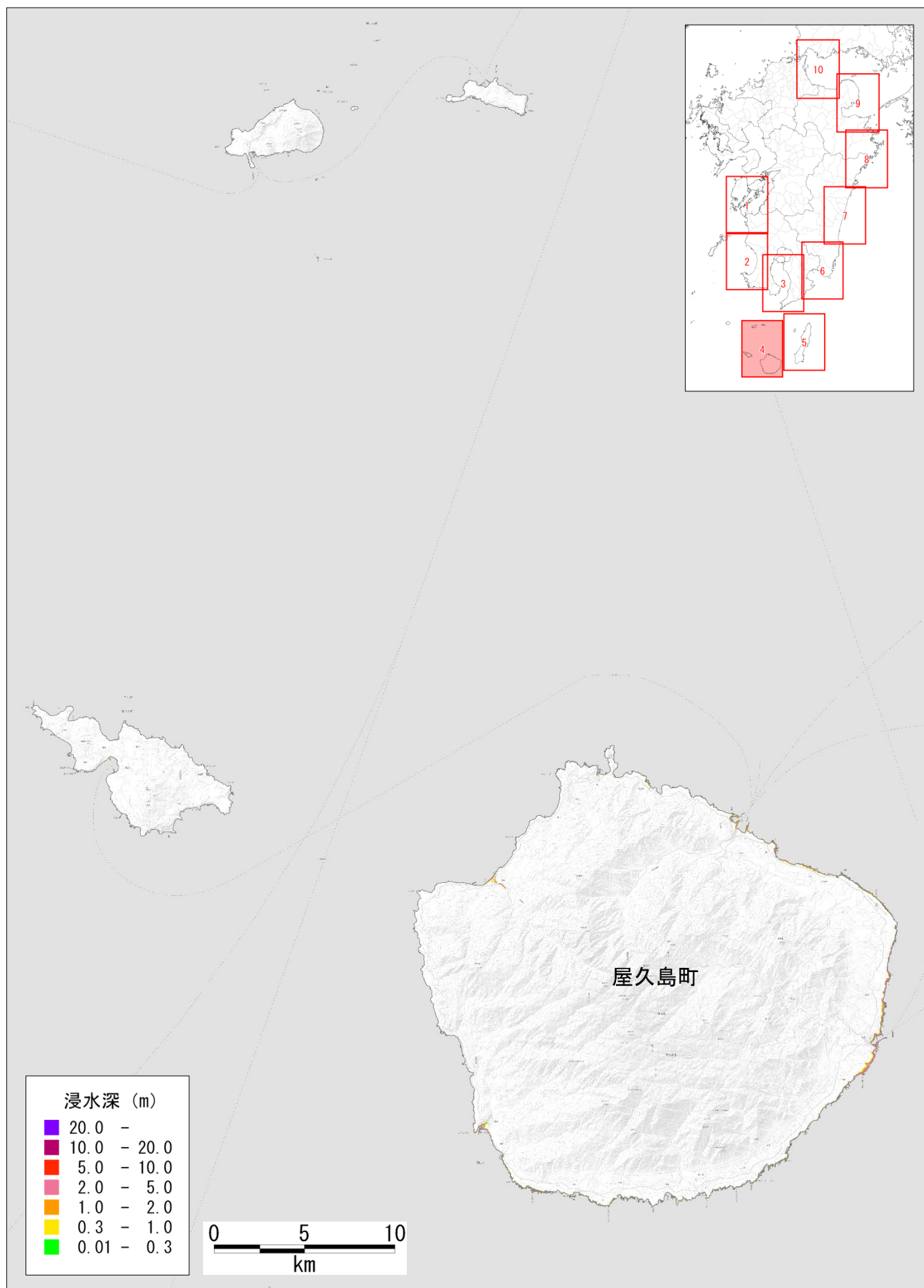
図 津波の浸水分布 【最大クラスケース③、堤防条件：津波が乗り越えたら破堤する】
