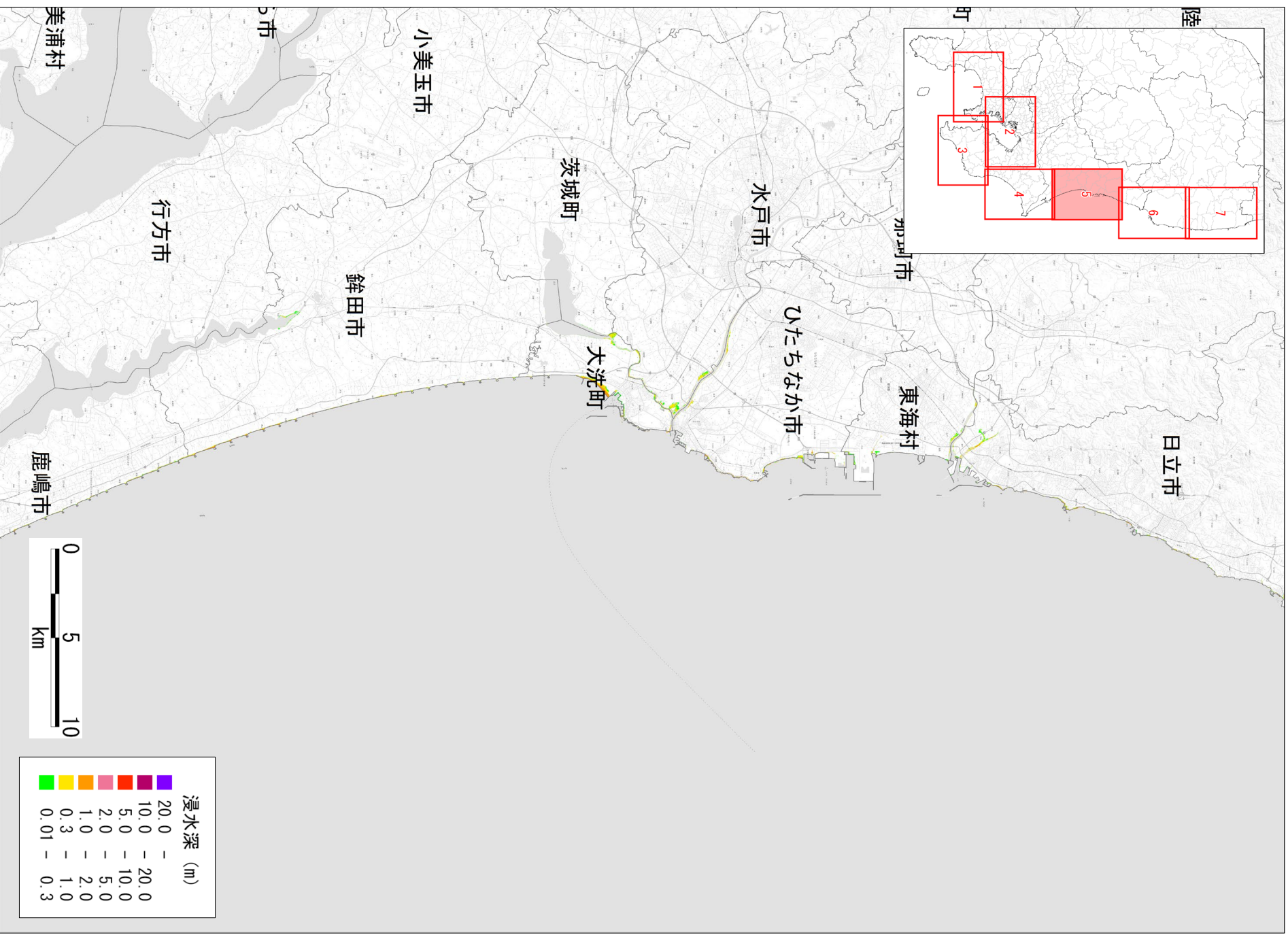
図 津波の浸水深分布
