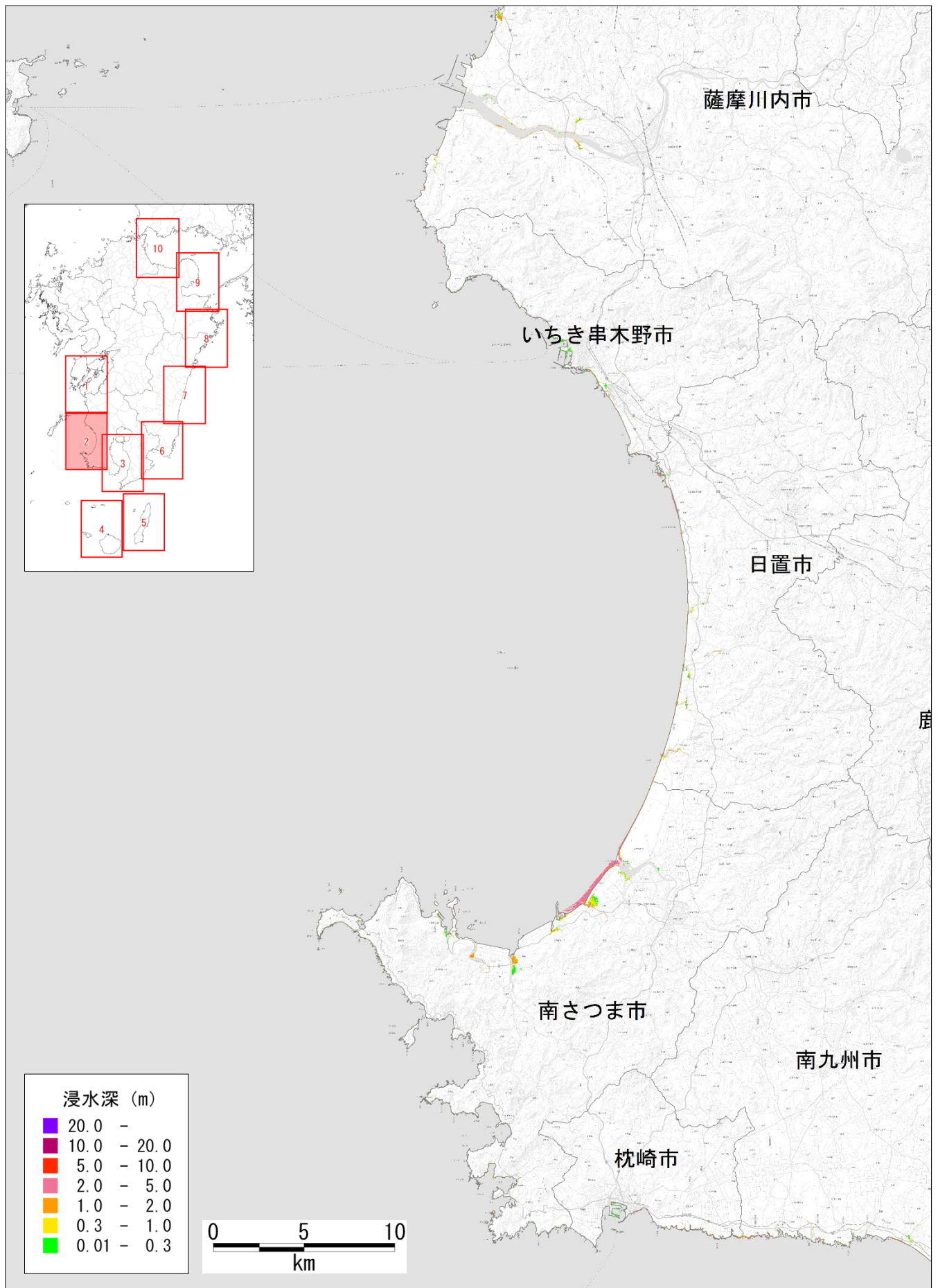
図 津波の浸水分布 【最大クラスケース③、堤防条件：津波が乗り越えたら破堤する】
