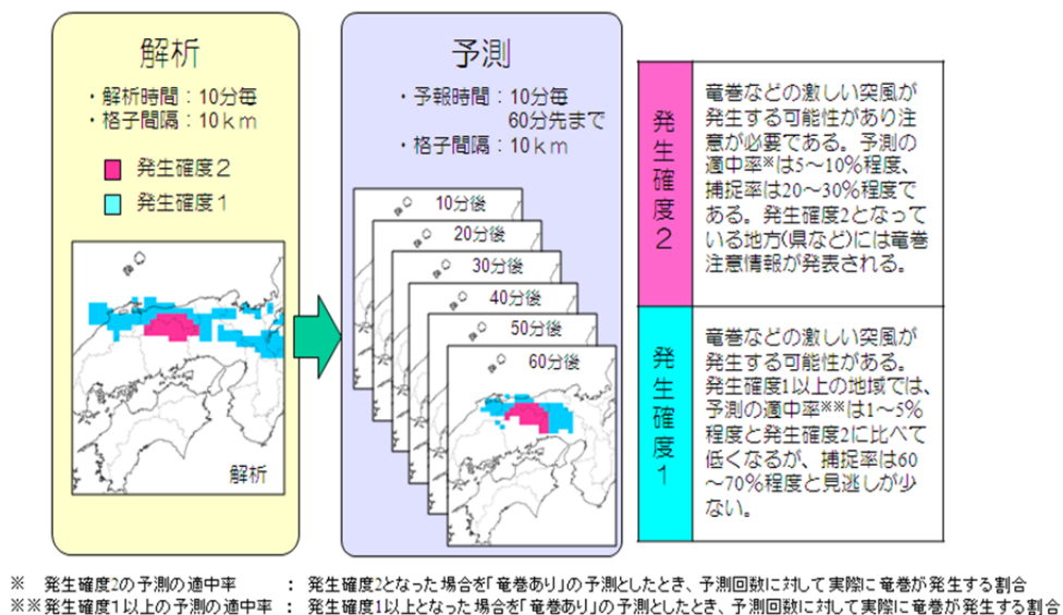
図表 3 竜巻発生確度ナウキャストについて
