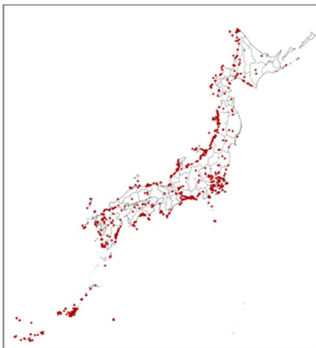
図表 11 分布図（全国）（1961～2010 年）
