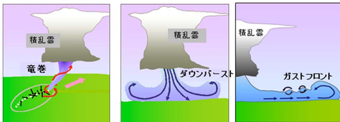
図表 12 竜巻、ダウンバースト、ガストフロントの概念図
