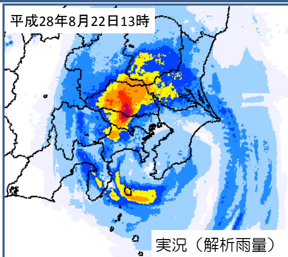
降水短時間予報の予測例（平成28年台風第9号）
