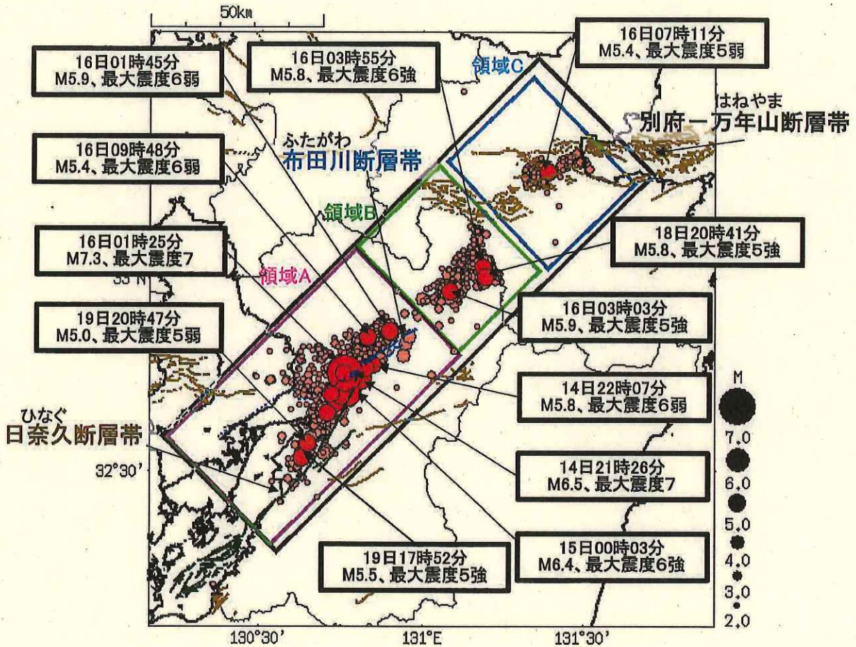
震央分布図
