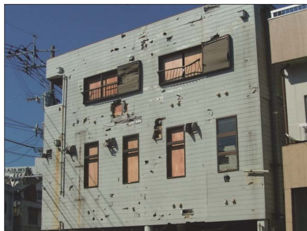
壁の全面にわたって飛来物による衝突痕、突き刺さり、貫通痕がある。
