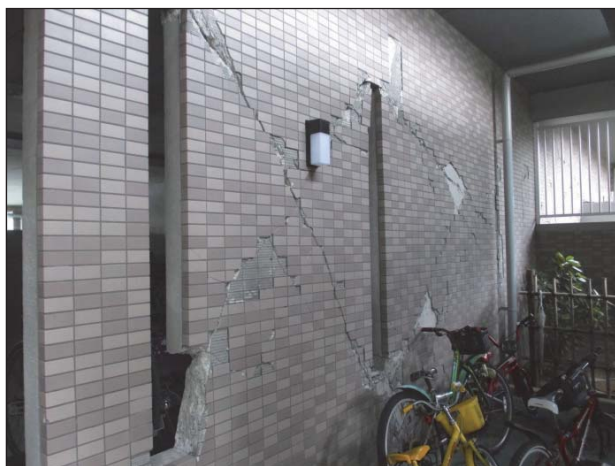
【雑壁】 全体にひび割れ(幅約0.2mm～1mm)やはがれが生じている。
