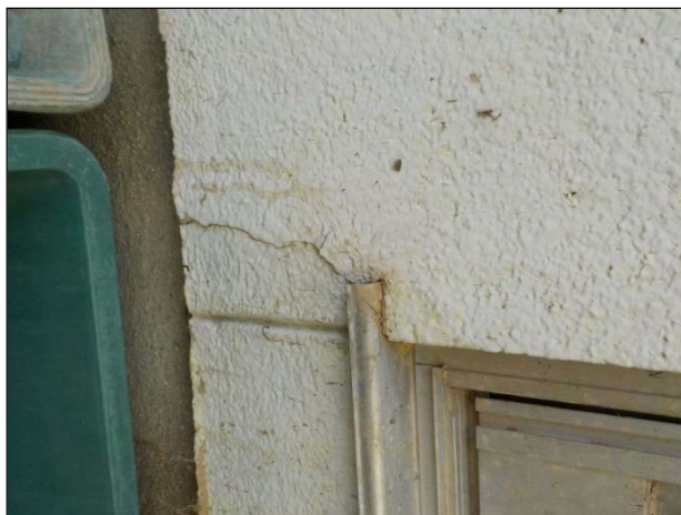
【モルタル塗り仕上等】 開口隅角部廻りにわずかなひび割れが生じている。
