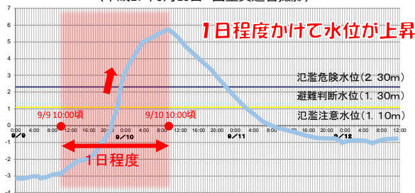
平成27年9月関東・東北豪雨災害時の鬼怒川の水位上昇
