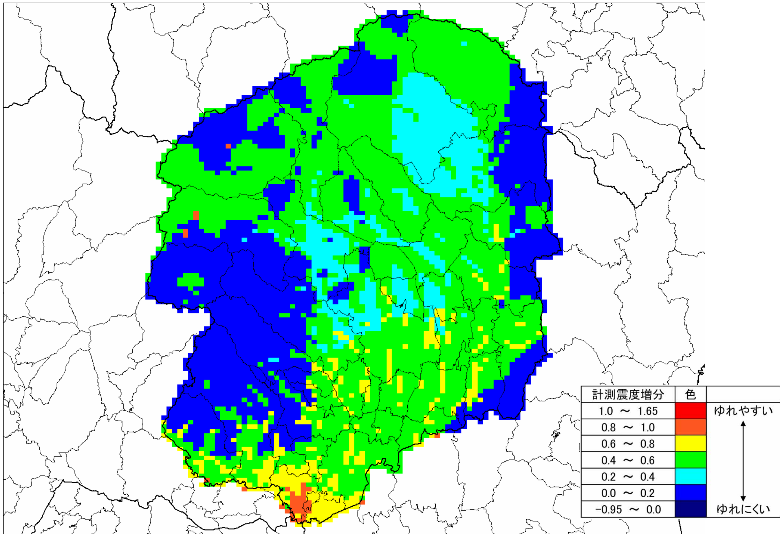
図 表層地盤のゆれやすさ（栃木県）
