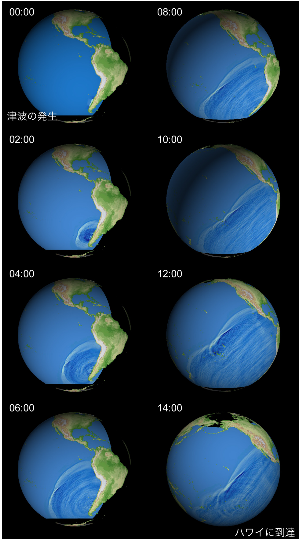
口絵 1 数値解析によるチリ地震津波の再現
