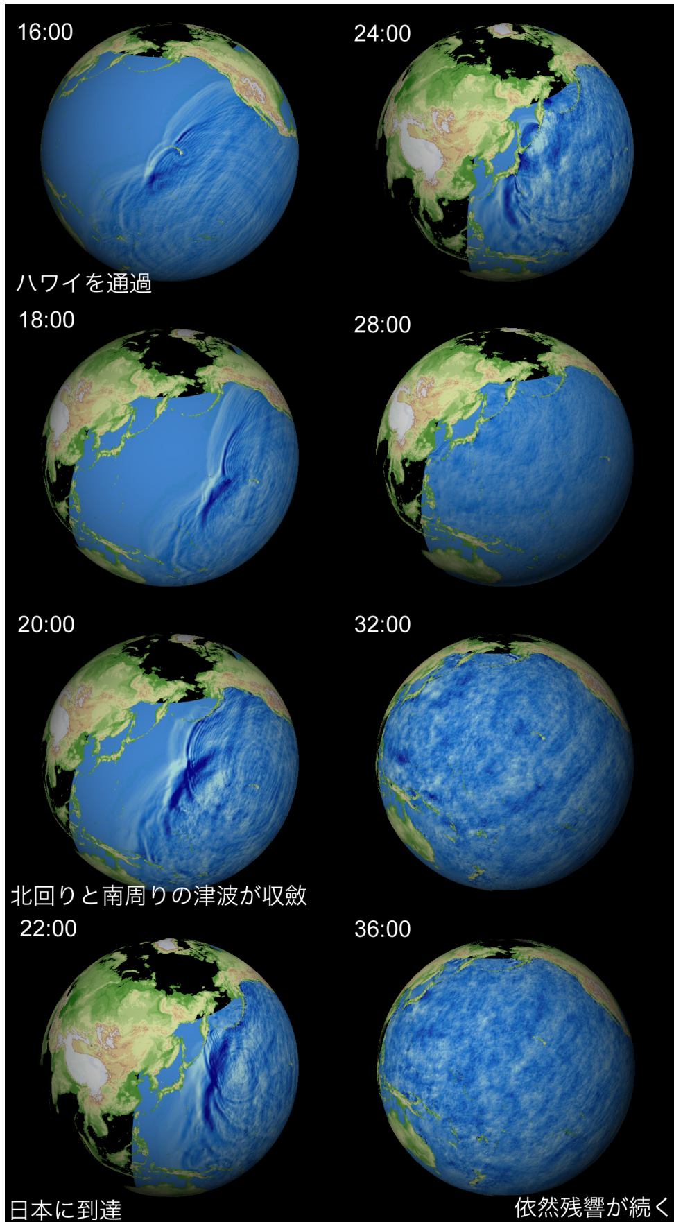
図2 数値解析によるチリ地震津波の再現
