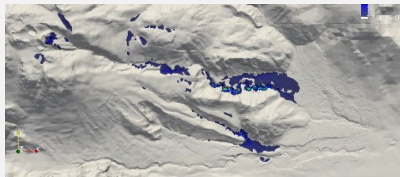
1991年雲仙普賢岳火砕流における数値計算による最終堆積物の分布
