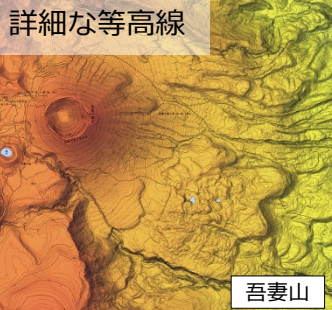
火山基本図
