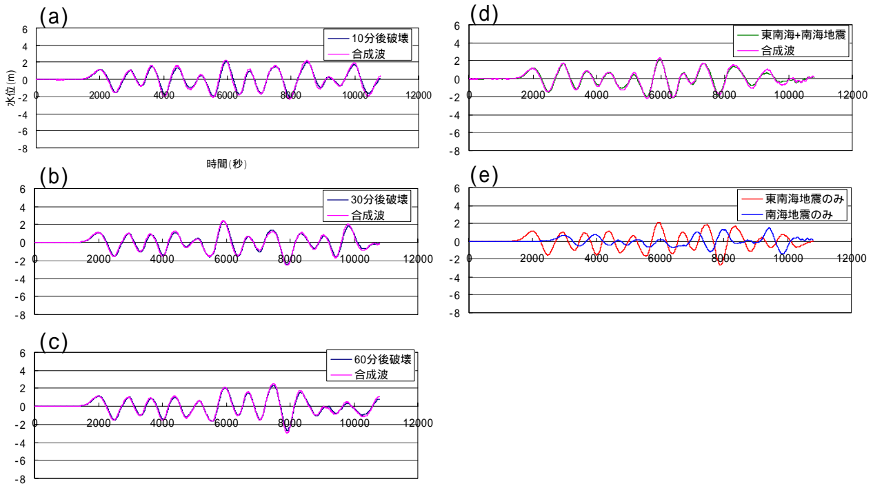
図 1-2 時間差を持って発生した場合の東南海・南海地震の水位波形と東南海地震の水位波形と南海地震の水位波形の合成波の比較（下田港）
