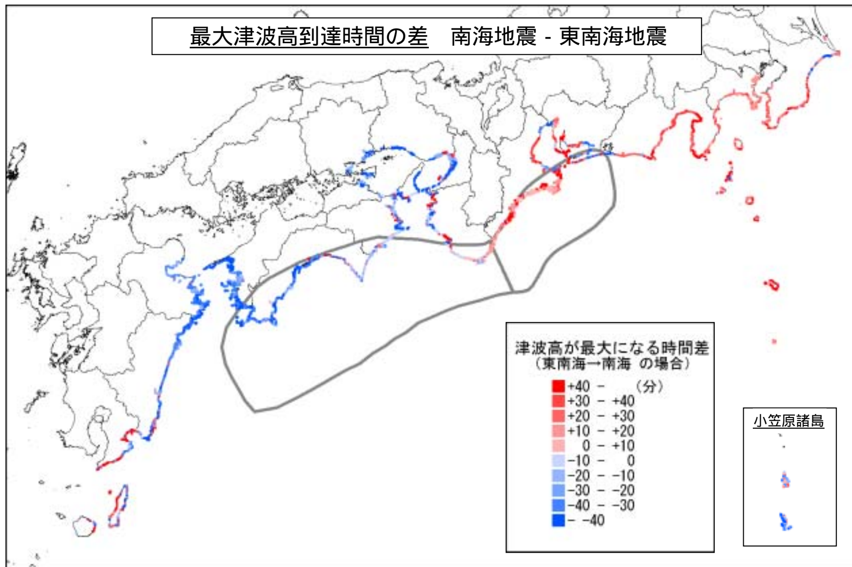
図 1-8 東南海地震の何分後に南海地震が発生すると各地の津波高が最大になるかを示す。その場合の津波高が 1 m 以上のメッシュのみ表示している。
