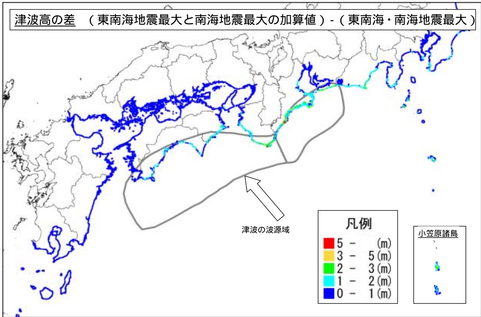
図 1-7 東南海地震の最大津波高と南海地震の最大津波高の加算値から東南海・南海地震の最大津波高を差し引いた高さ。東南海領域と南海領域が時間差をもって発生する場合に、東南海・南海地震よりも大きくなる津波高の最大値を示す。
