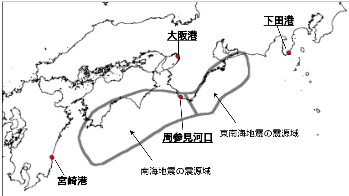
図 1-1 断層モデルと水位波形出力地点の位置
