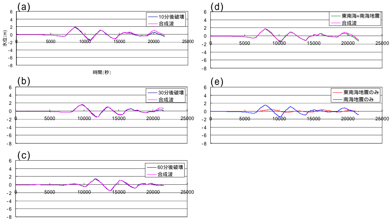
図 1-4 時間差を持って発生した場合の東南海・南海地震の水位波形と東南海地震の水位波形と南海地震の水位波形の合成波の比較（大阪港）
