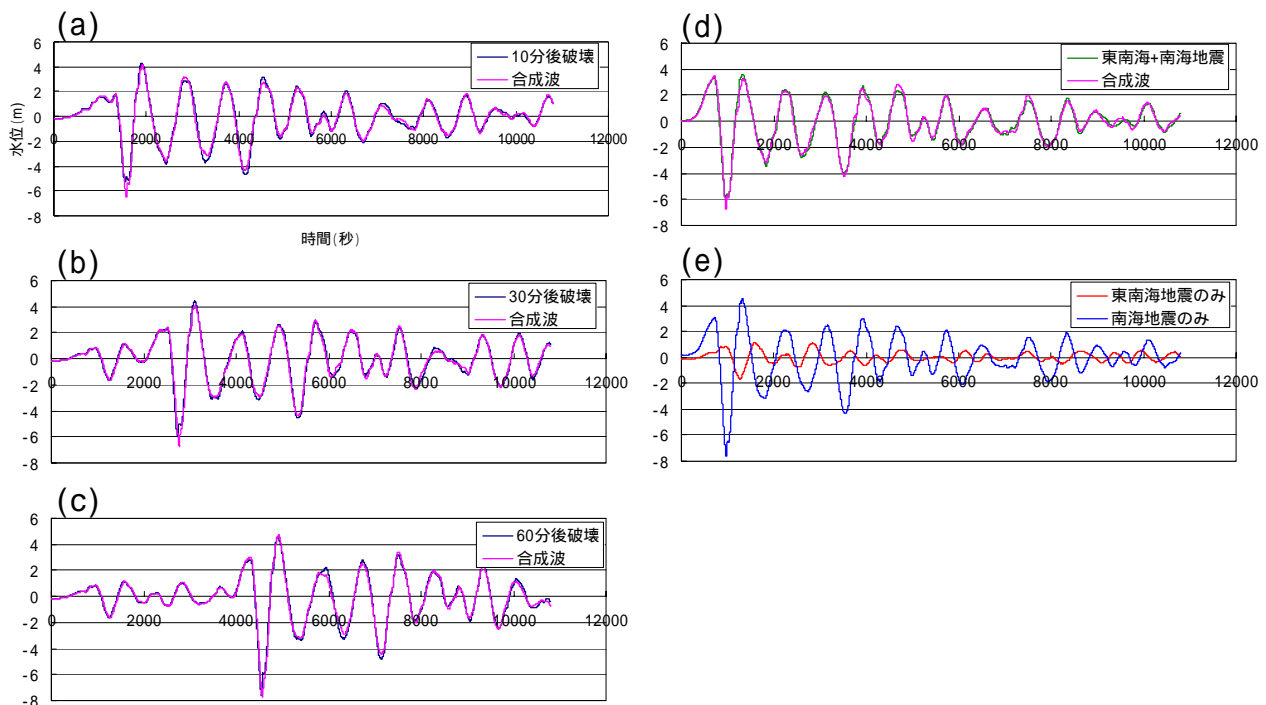
図 1-3 時間差を持って発生した場合の東南海・南海地震の水位波形と東南海地震の水位波形と南海地震の水位波形の合成波の比較（周参見河口）
