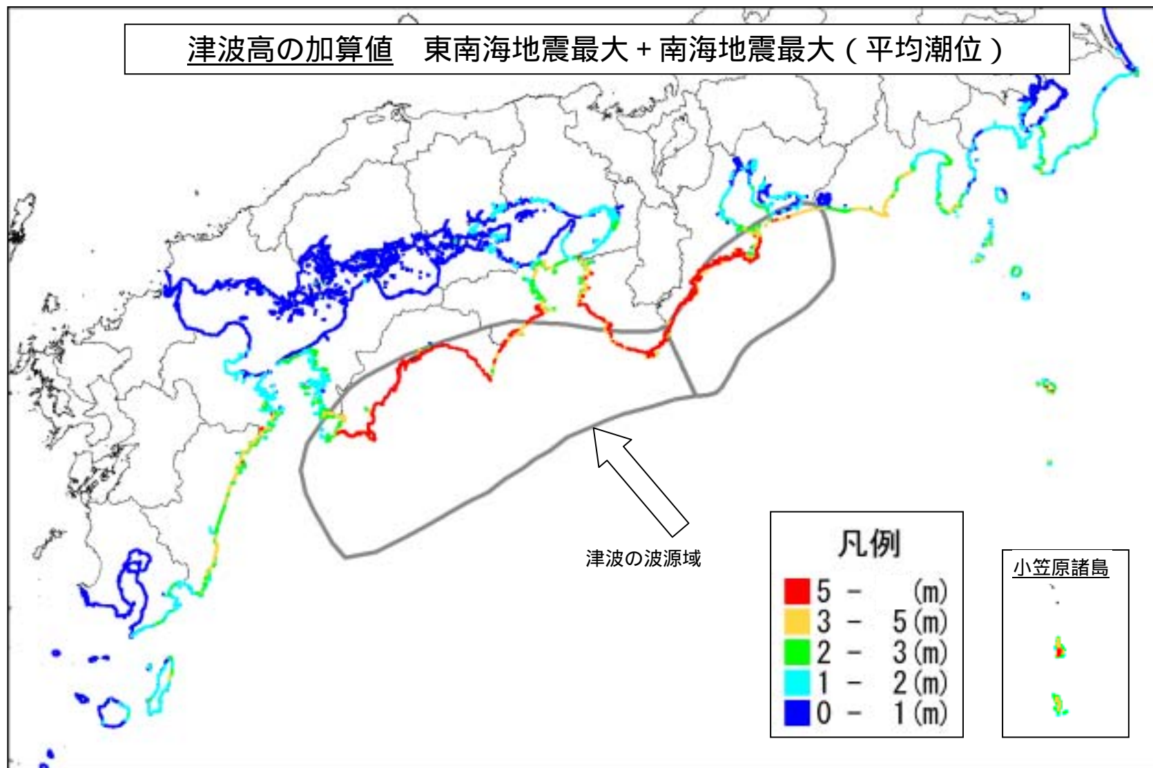
図 1-6 東南海地震の最大津波高と南海地震の最大津波高の加算値。東南海領域と南海領域が時間差をもって発生する場合の各地の津波高の最大値を示す。
