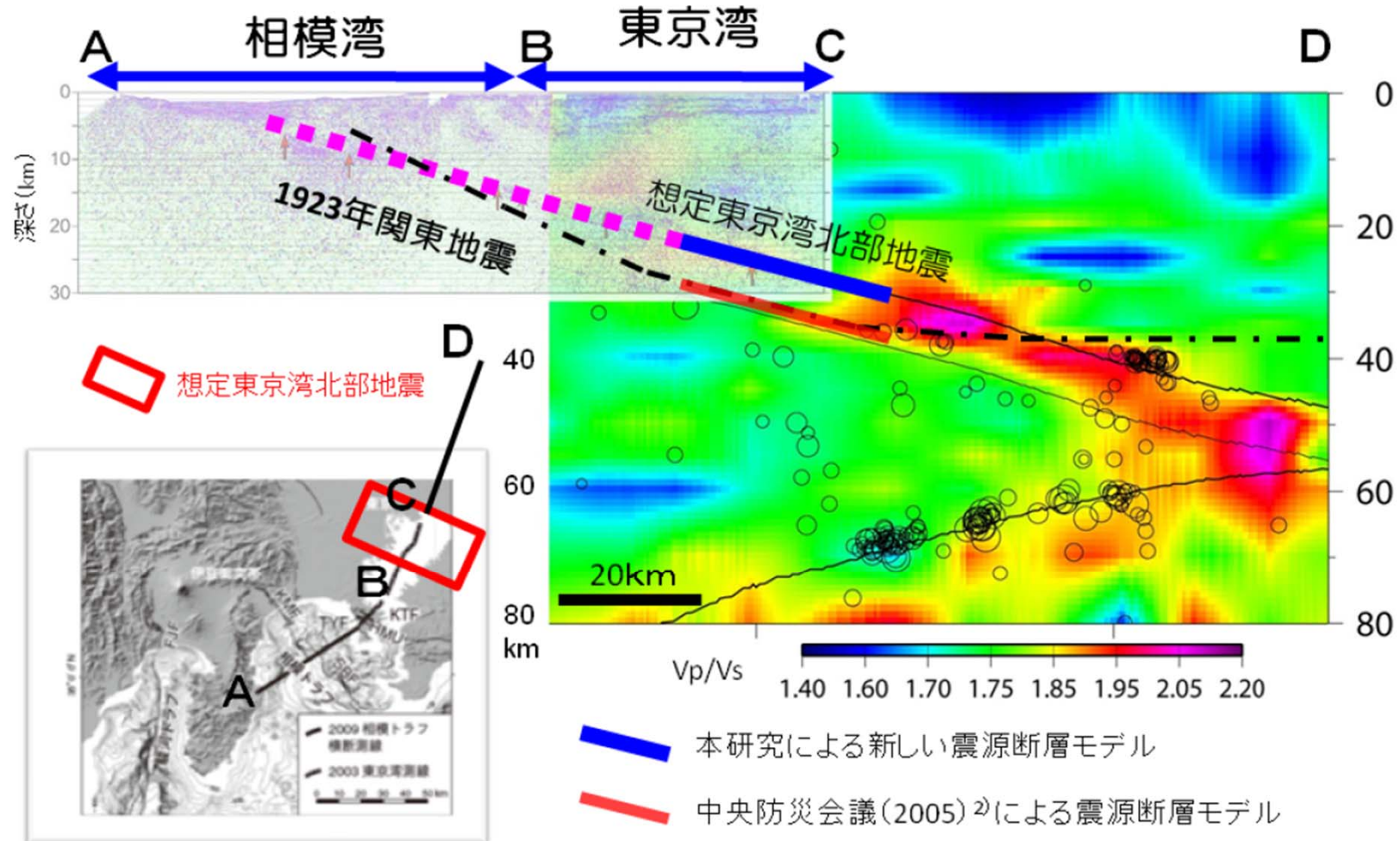
図 想定された東京湾北部の地震断層面の深さの比較。中央防災会議が想定した地震断層面(赤)と、本プロジェクトによる震源断層面(青)。反射法地震探査断層面図と V_p/V_s の分布をあわせて示し、Ishida(1992)による古いプレートモデルを一点鎖線で、1923年関東地震の震源断層面を破線で示しました。東京湾北部の地震断層面は、これまでの結果より約10km浅くなり、その周辺の陸の下部地殻やPHSプレートの海洋性地殻の V_p/V_s が標準的な値を示す領域(緑色)に位置するため、地震を起こさない領域であるとは言えません。
