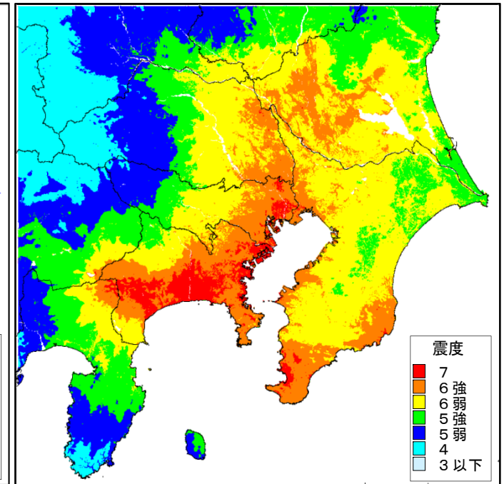
相模トラフ沿いの最大クラスの地震の震度分布 (M8クラス) Mw8.7
