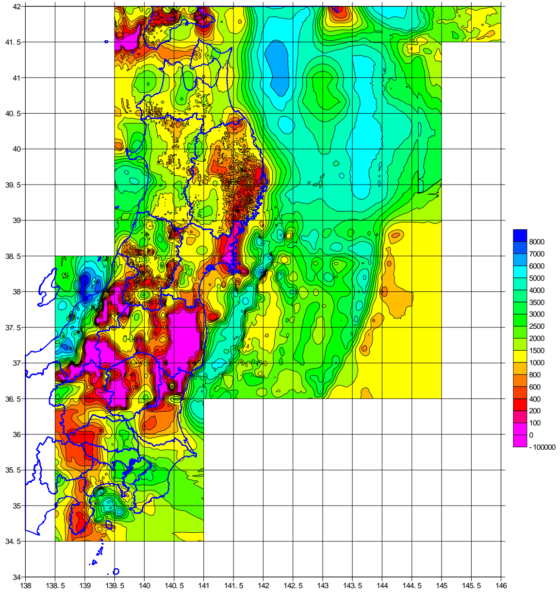
図 8 - 1 0 ( 5 ) S 波速度 2.4km/s 層上面深度 ( 関東地方から東北地方 )
