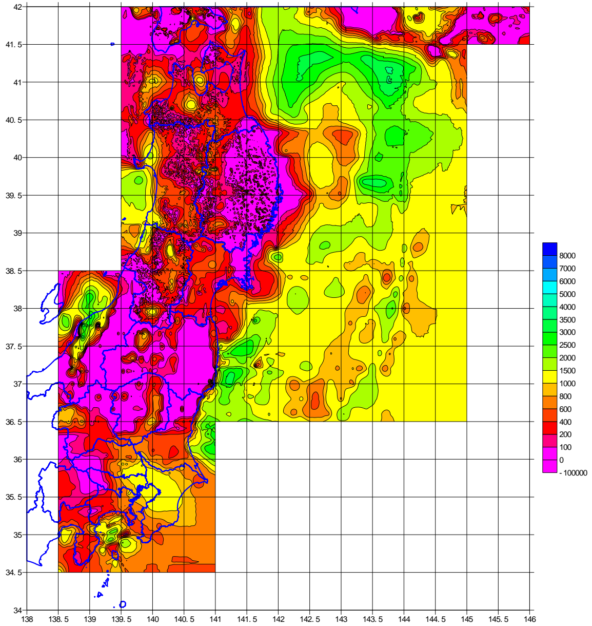
図 8 - 1 0 ( 2 ) S 波速度 1.0km/s 層上面深度 ( 関東地方から東北地方 )
