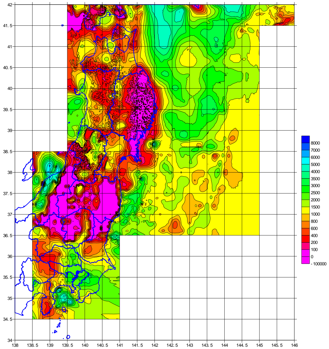
図 8 - 1 0 ( 4 ) S 波速度 2.1km/s 層上面深度 ( 関東地方から東北地方 )
