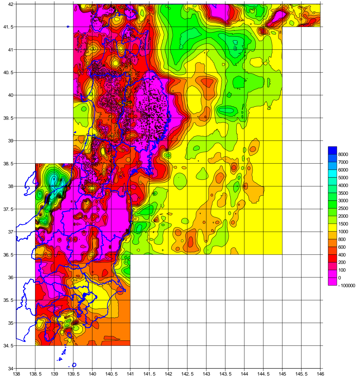
図8 - 10 ( 3 ) S波速度 1.4km/s 層上面深度 ( 関東地方から東北地方 )
