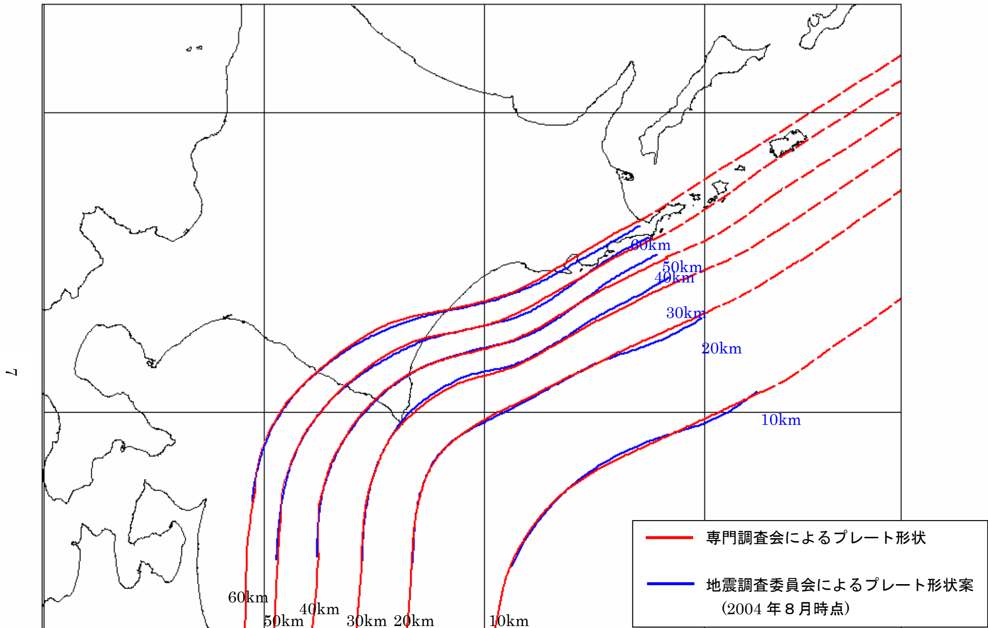
図 1-7 専門調査会と地震調査委員会によるプレート形状案
