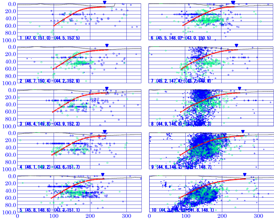
図1-6 プレート形状の断面図 赤色実線はプレート形状、青色▼は海溝軸の位置 青色●は気象庁震源、緑色●はNEIC震源 (M4.5以上) 黒色実線は海底面、緑色実線は地表面
