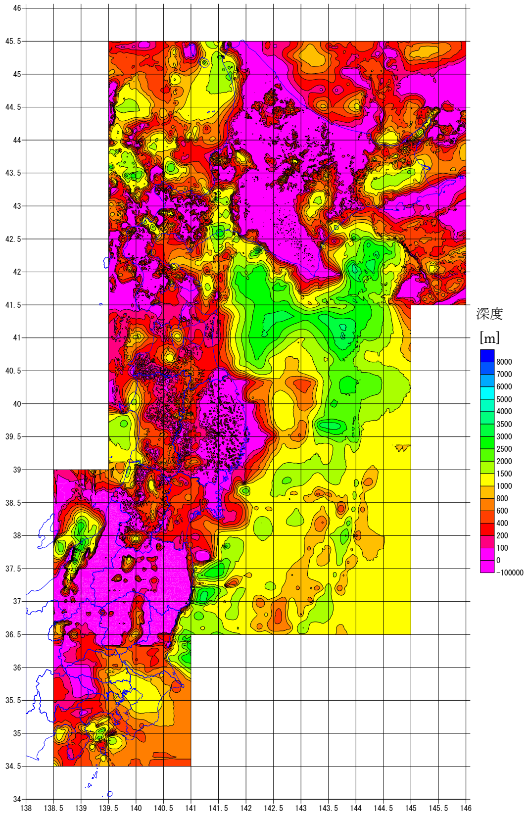
图 2. 1 9 P 波速度 2.5km/s 程度層 上面深度図
