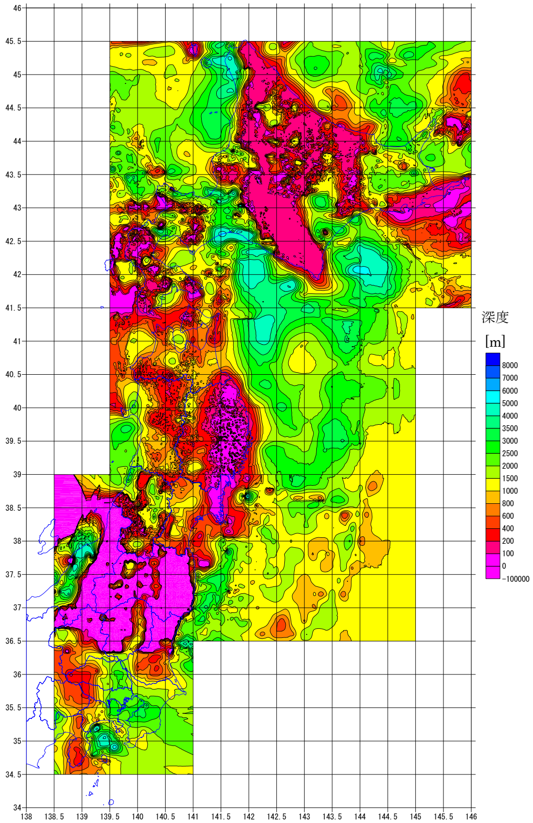
图 2. 1 7 P 波速度 4.0km/s 程度層 上面深度図
