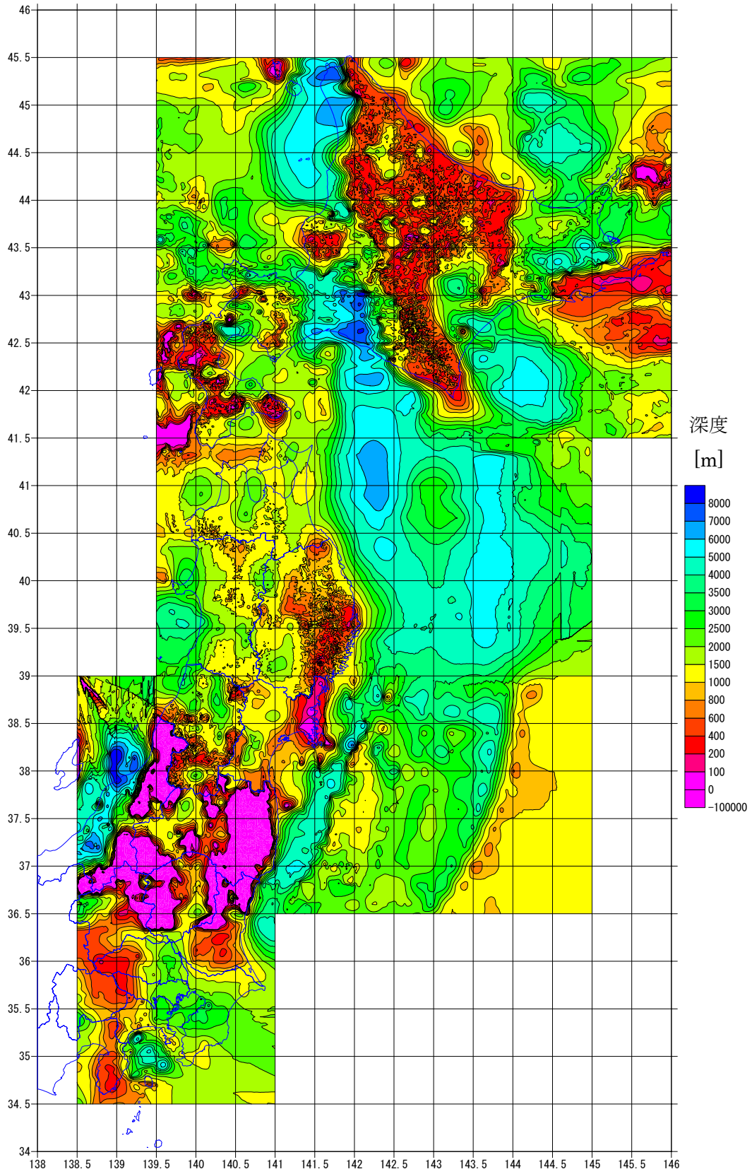
图 2. 16 P 波速度 4.8km/s 程度層 上面深度図
