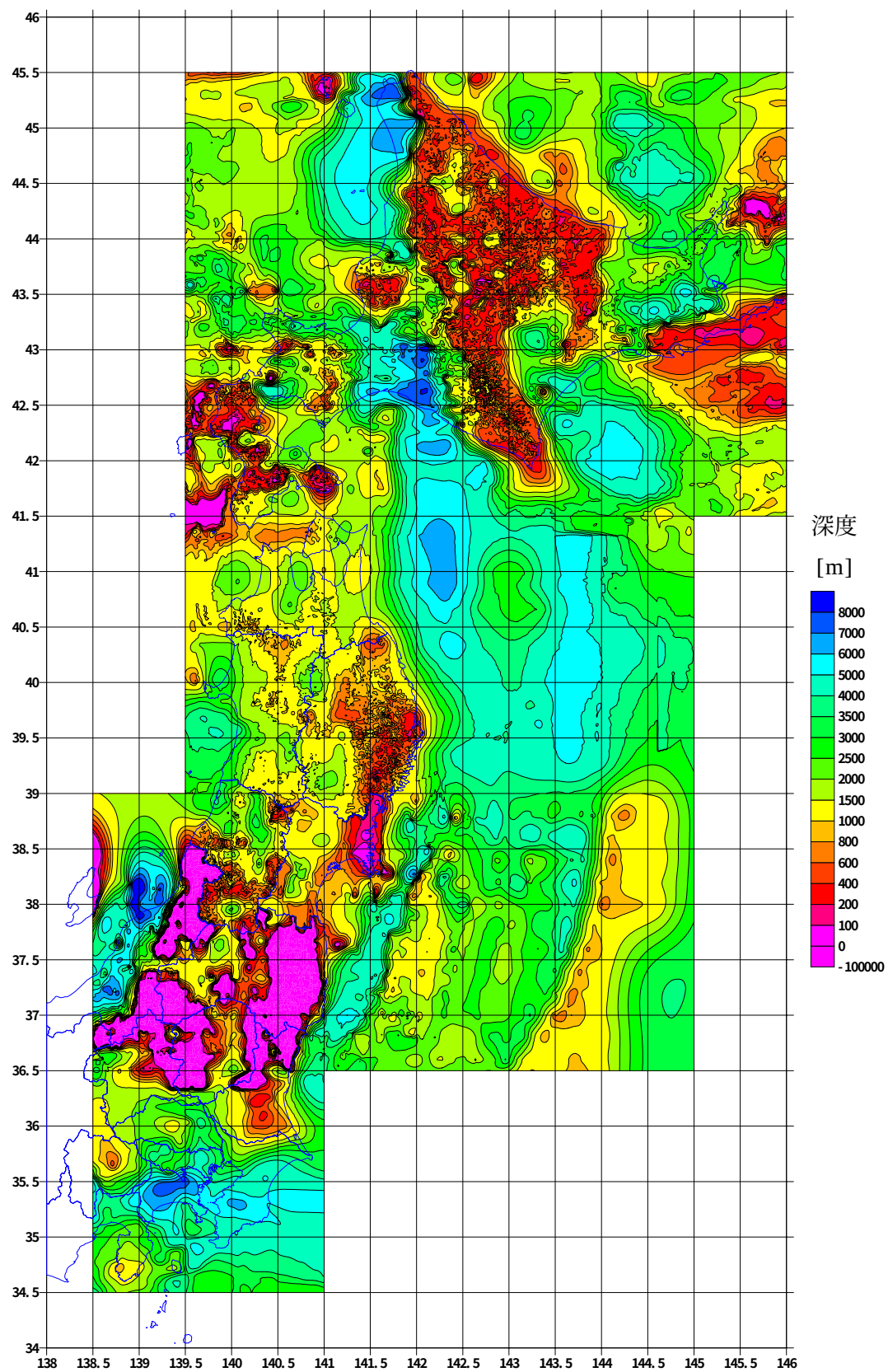
图2. 15 P波速度5.5km/s程度層 上面深度図
