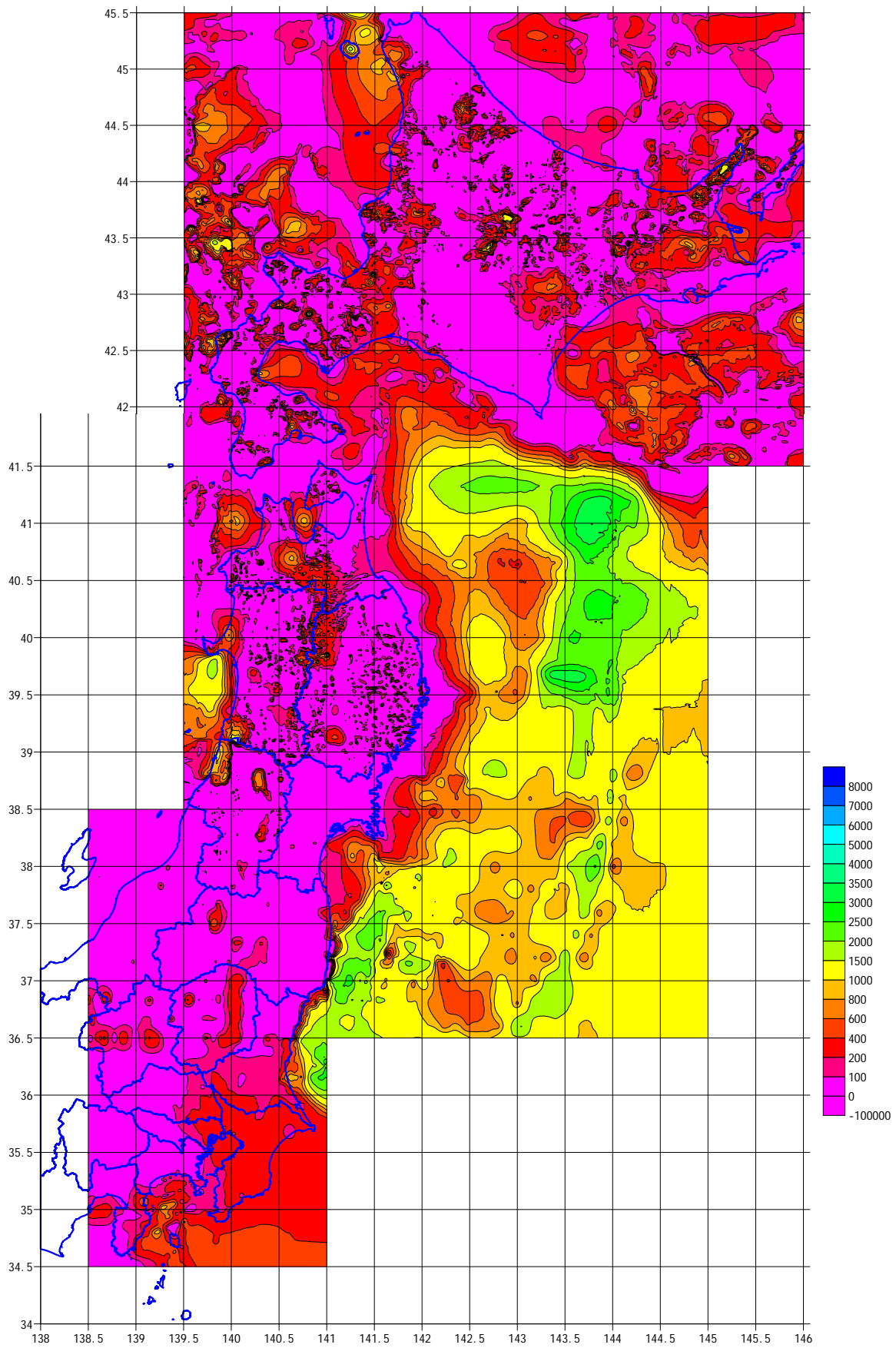
图 2-1-5 S 波速度 0.7km/s 層上面深度
