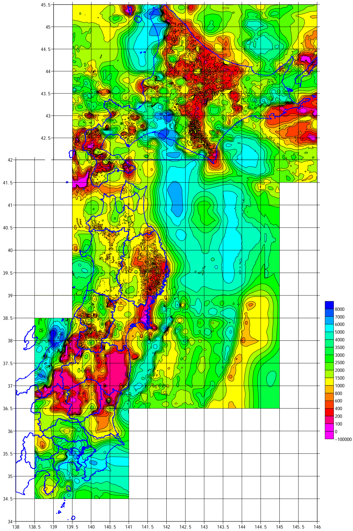
图 2-1-6 S 波速度 3.0km/s 層上面深度
