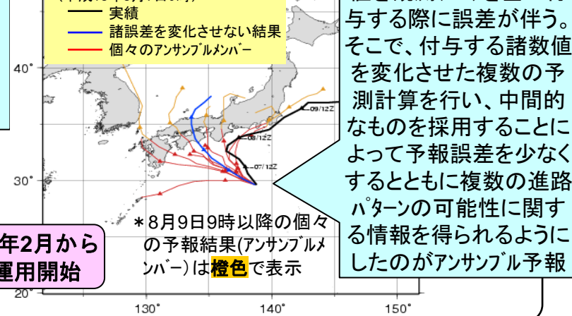
台風EPSの進路予報例 (平成18年8月7日9時)
