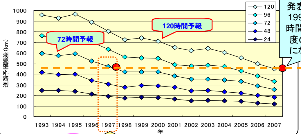
全球モデル台風進路予報誤差(3年移動平均)
