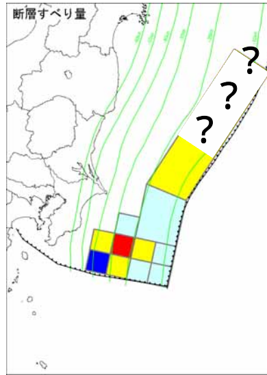
図 3-3-10-4 1677年延宝房総沖の地震インバージョン：断層モデルおよび遡上高（平均潮位）
